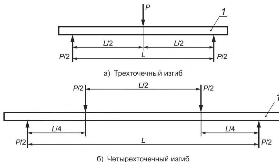
Рисунок 2 — Виды нагружения образца
