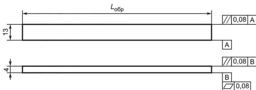
Рисунок 1 — Образец для испытаний
