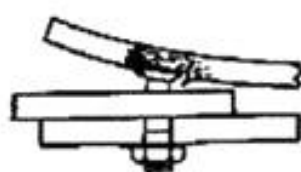
PLT (протягивание ламината, отверстие в ламинате, вверху)
