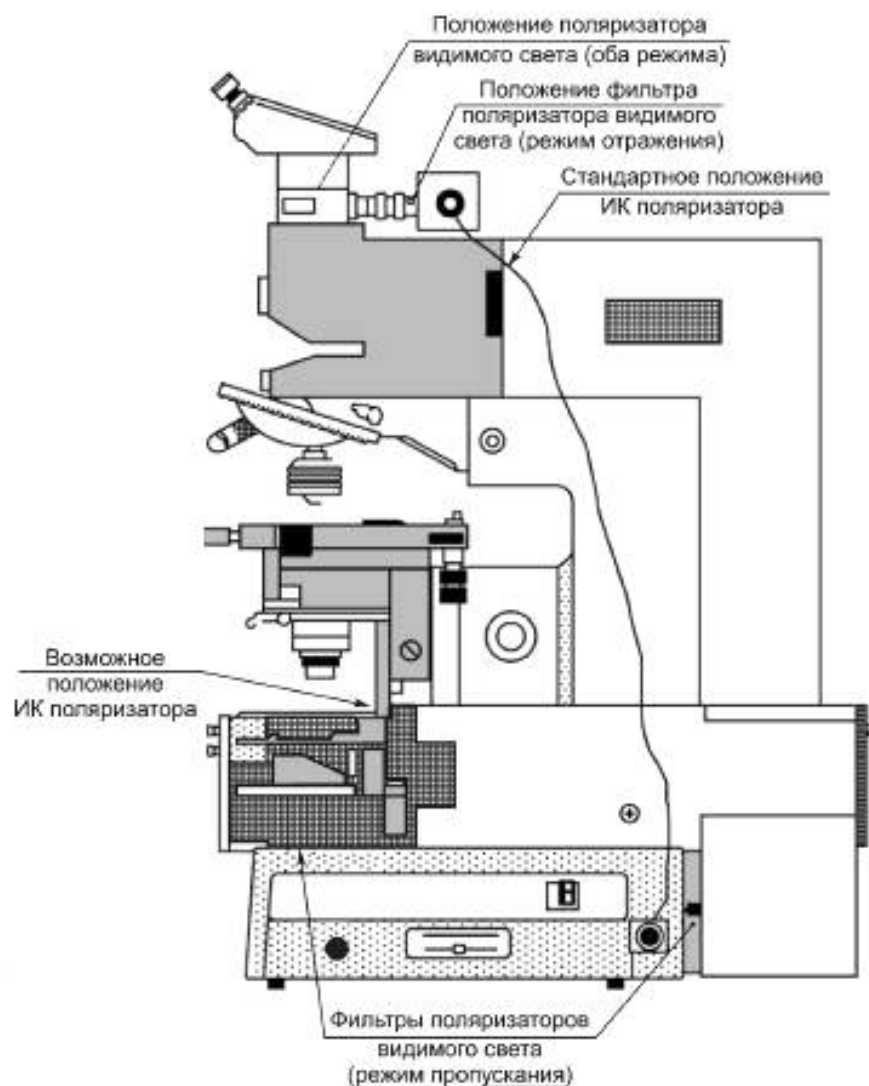
Рисунок 3 — Упрощенная схема приспособления для инфракрасной микроскопии
