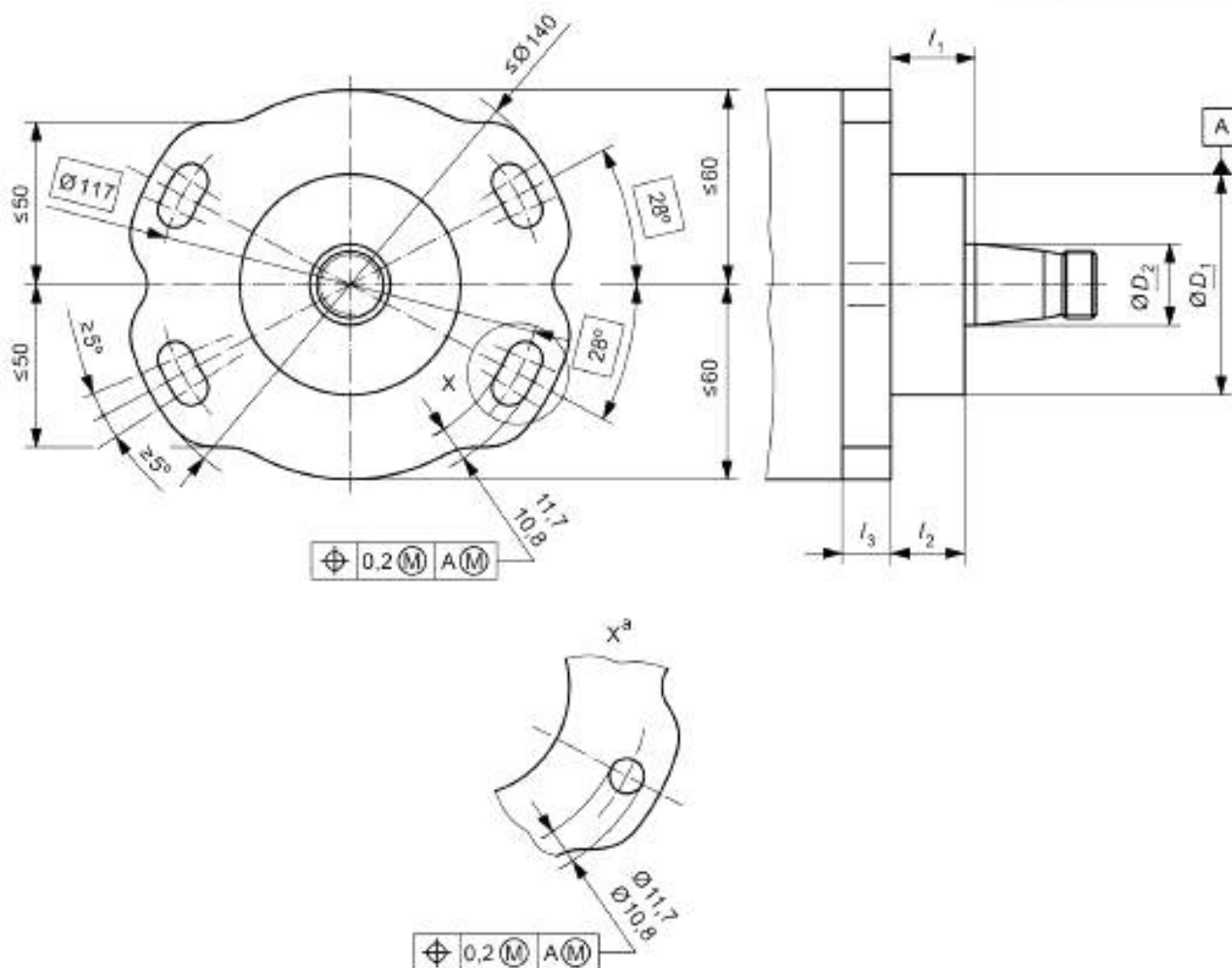
Рисунок 9 — Монтажный фланец типа 9
