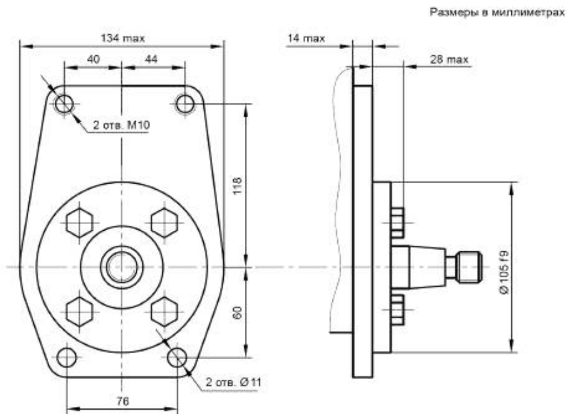
Рисунок 10 — Монтажный фланец типа 10
