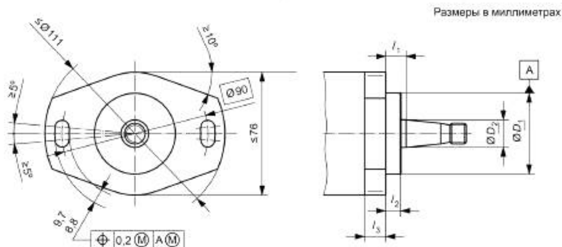
Рисунок 1 — Монтажный фланец типа 1
