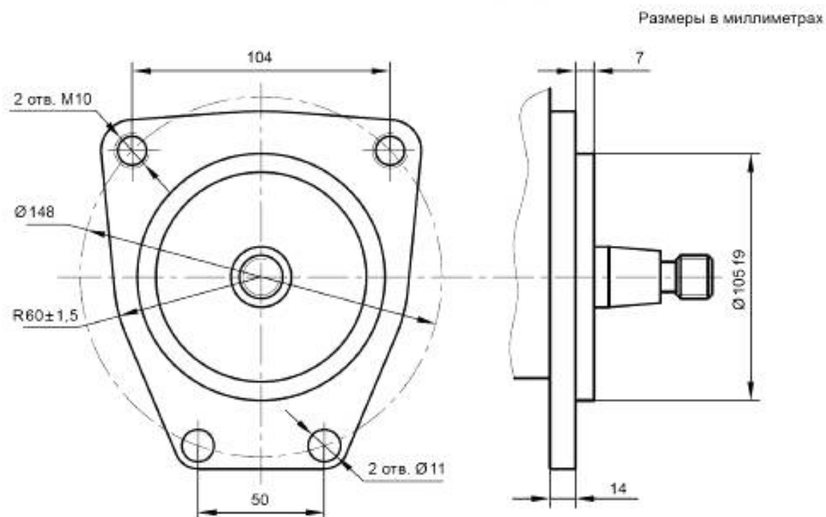
Рисунок 11 — Монтажный фланец типа 11
