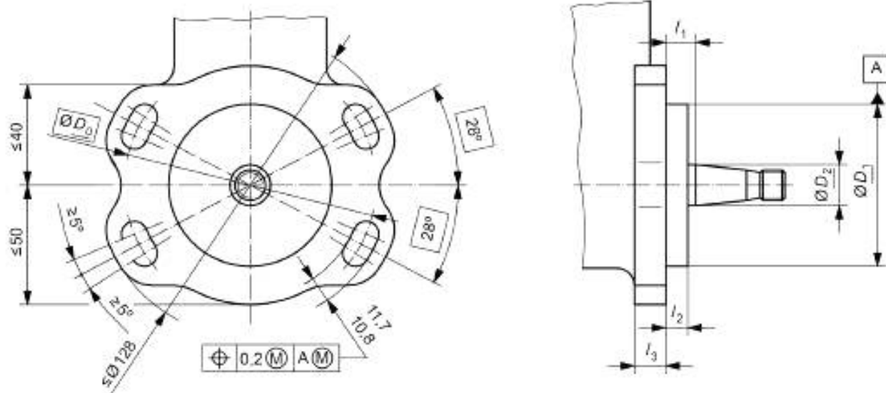
Рисунок 7 — Монтажный фланец типа 7
