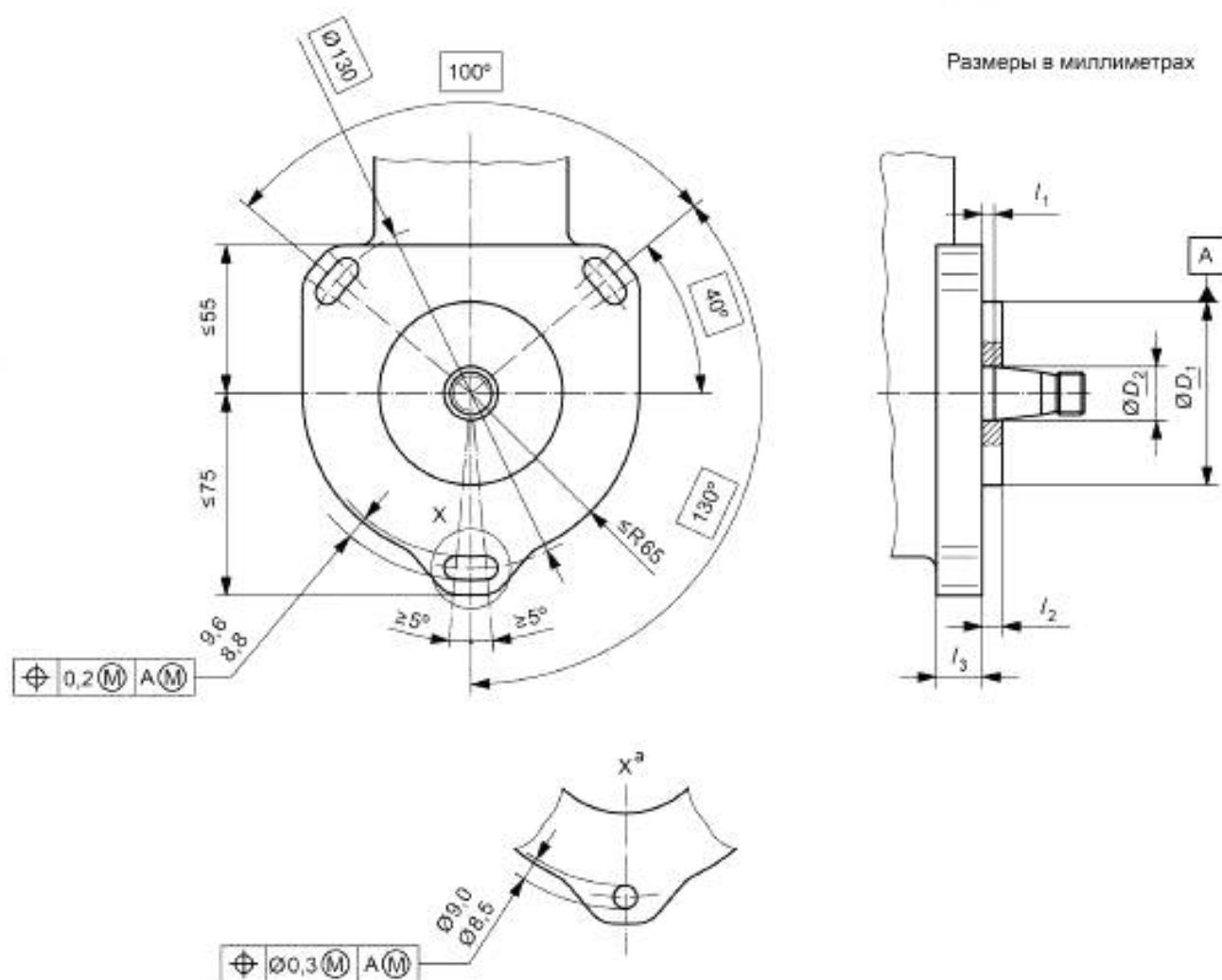
Рисунок 6 — Монтажный фланец типа 6
