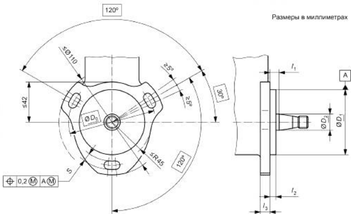
Рисунок 4 — Монтажный фланец типа 4
