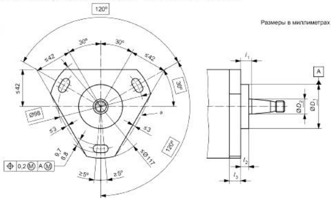
Рисунок 2 — Монтажный фланец типа 2
