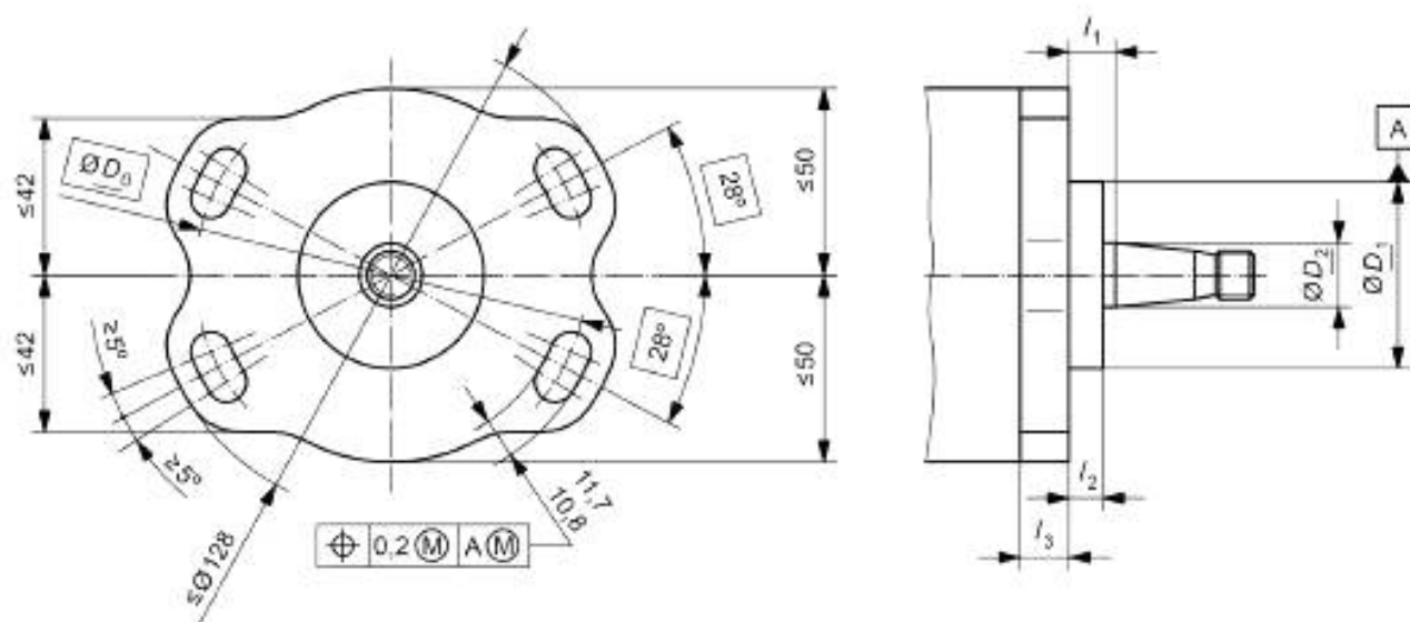
Рисунок 3 — Монтажный фланец типа 3
