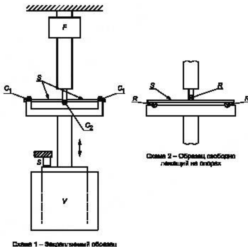
Рисунок 1 — Возможные схемы устройства нагружения для определения динамических модулей при изгибе
