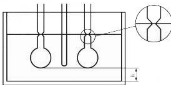
Рисунок 2 — Схема погружения измерительной системы вискозиметра в образец
