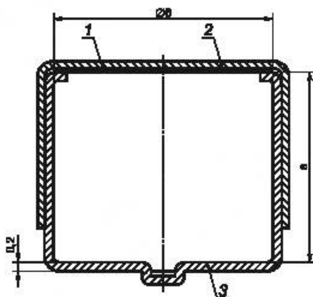
1 — уплотнитель; 2 — крышка; 3 — тигель
