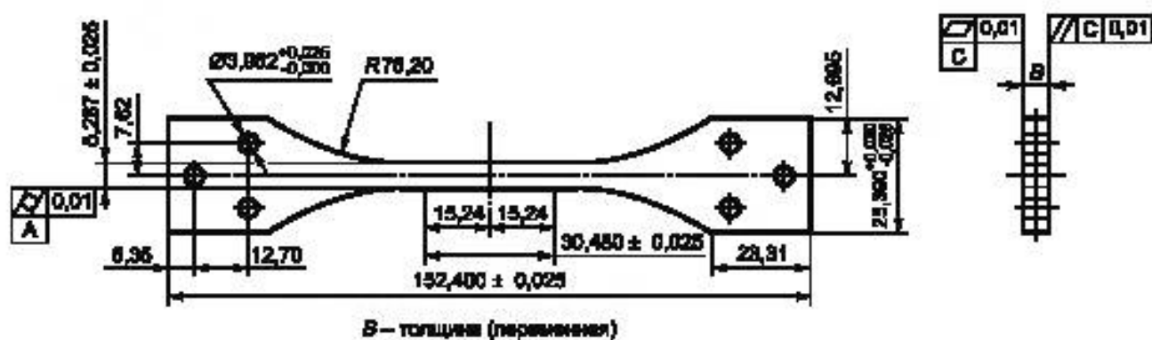
Рисунок 7 — Образец типа VII
