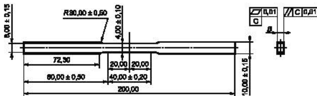
Рисунок 5 — Образец типа V
