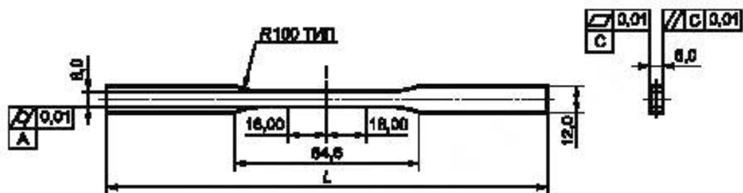
Рисунок 6 — Образец типа VI
