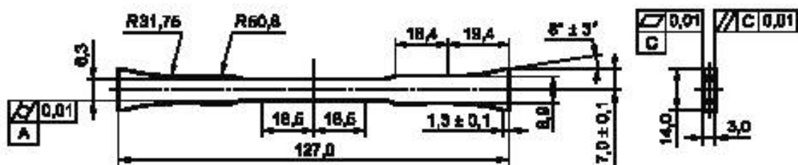
Рисунок 3 — Образец типа III
