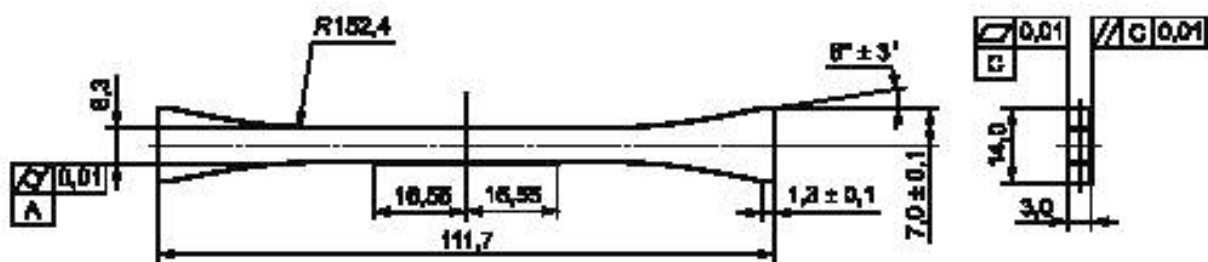
Рисунок 2 — Образец типа II
