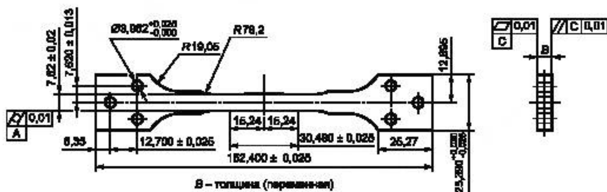
Рисунок 8 — Образец типа VIII
