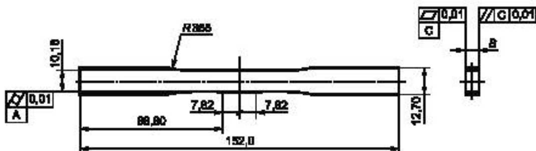
Рисунок 3 — Образец типа III
