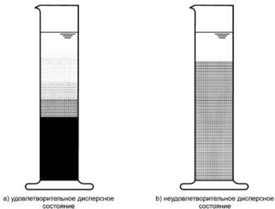
Рисунок 1 — Оценка дисперсного состояния пробы по процессу седиментации
