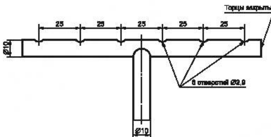
Рисунок А.9 — Горелка для калибровки
