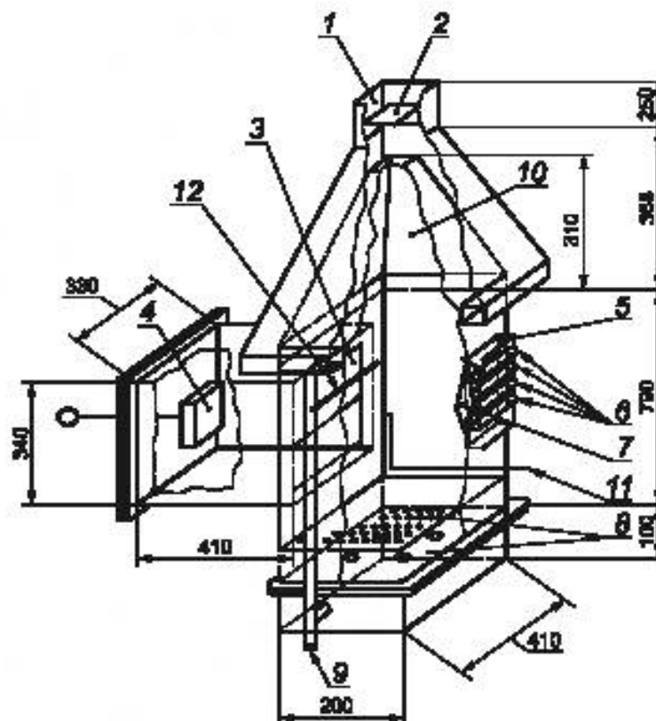
1 — дымовая труба; 2 — пластина; 3 — радиационные створки (в закрытом положении); 4 — держатель образца; 5 — панель источника теплового излучения; 6 — нагревательные стержни; 7 — маска для выравнивания теплового потока; 8 — воздухо-распределительные пластины; 9 — вход воздуха; 10 — воздухо-распределительный короб; 11 — нижняя запальная горелка; 12 — верхняя запальная горелка
