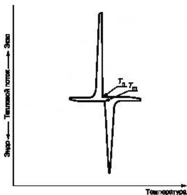
Рисунок 1 — Температуры плавления и кристаллизации чистого кристаллического материала
