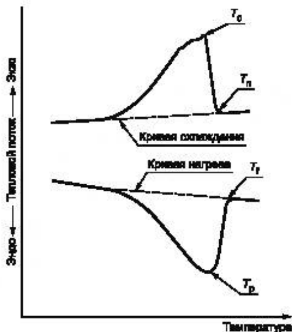
Рисунок 2 — Температуры плавления и кристаллизации полимерного материала
