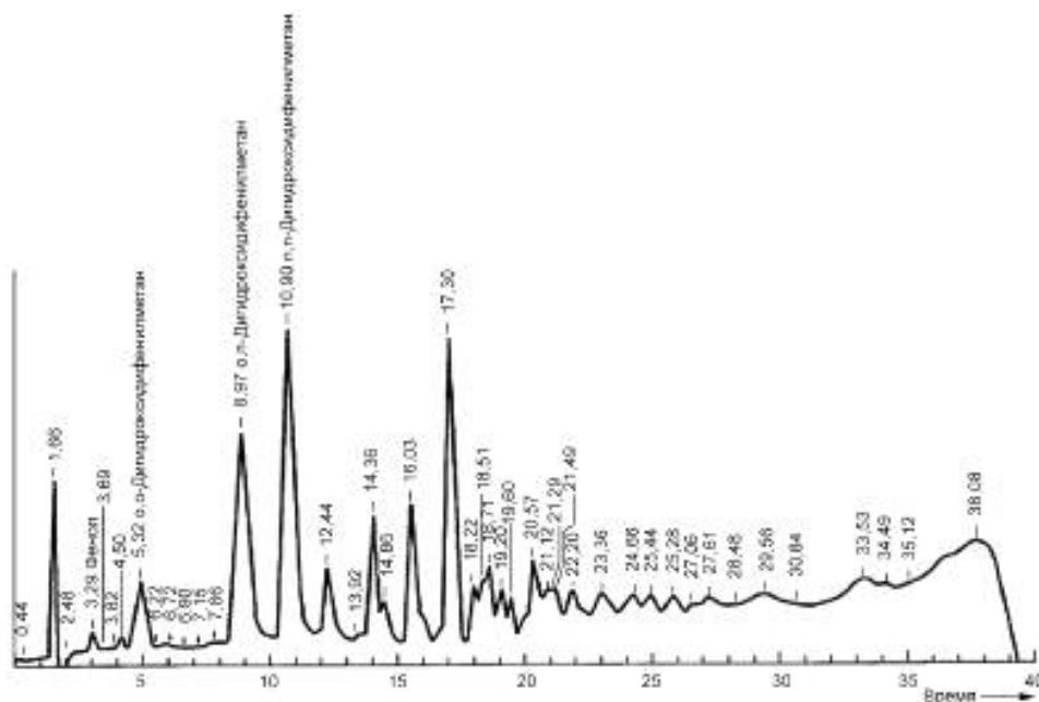
Рисунок 2 — Пример хроматограммы образца новолака на полярной колонке
