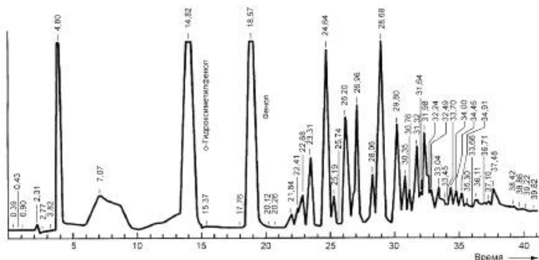
Рисунок 3 — Пример хроматограммы образца новолака на неполярной колонке
