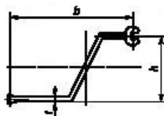
Рисунок 2 — Поперечное сечение зетовых композитных шпунтов
