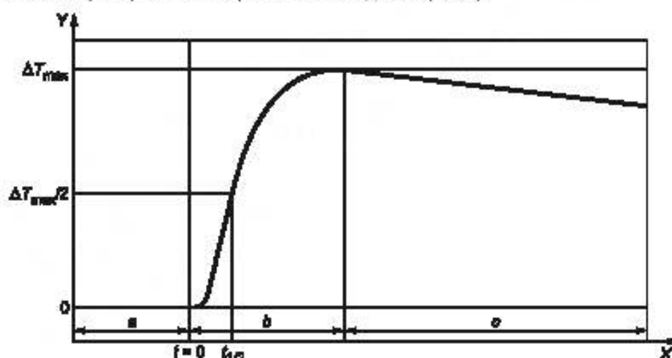
Рисунок 1 — Пример термограммы
