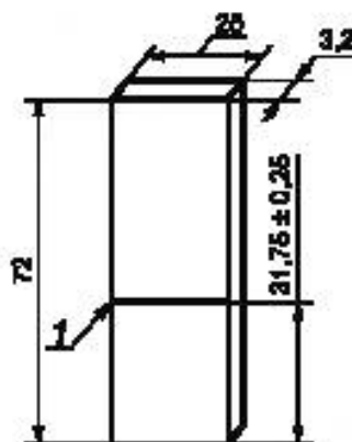
1 — обработанная машинным способом канавка, 0,8 мм
