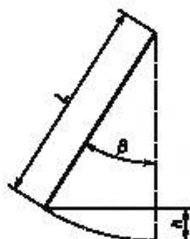
Рисунок В.1 — Взмах маятника из положения покоя
