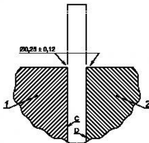
1 — неподвижная губка захватов; 2 — подвижная губка захватов
