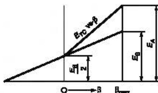
Рисунок В.2 — Полная поправка энергии на снос маятника и трение циферблата как функция от положения маятника
