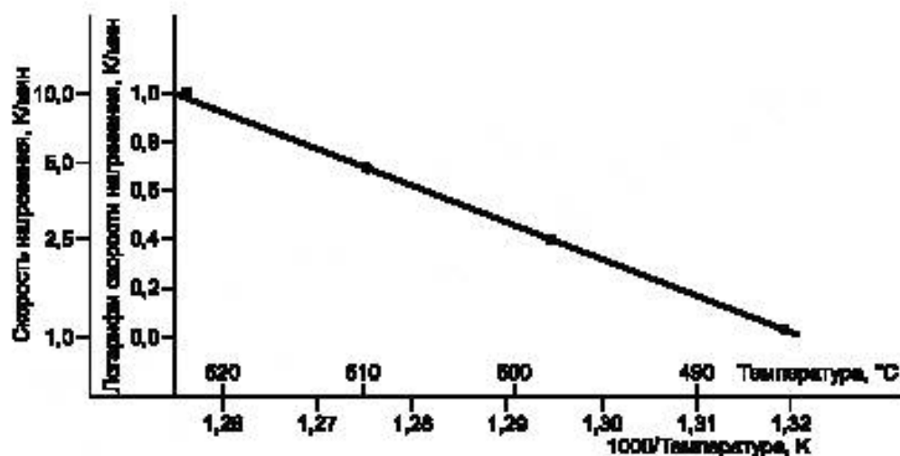
Рисунок 2 — График в координатах Аррениуса для скорости нагрева и температуры для данных постоянной степени превращения
