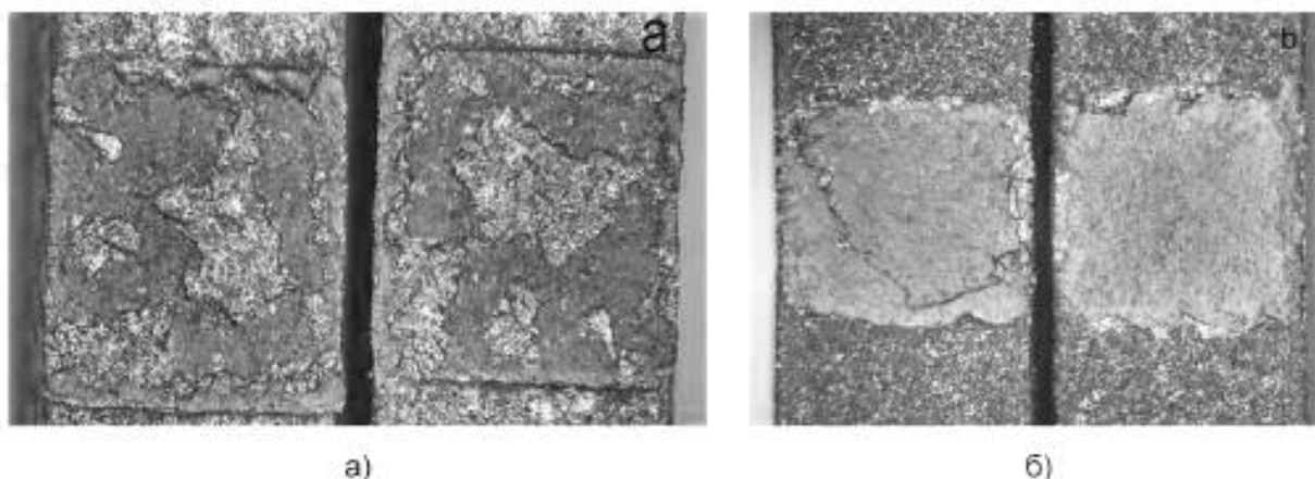
Рисунок 7 — Зона оксидного соединения крестообразных образцов \text{Ti}_3\text{SiC}_2 — \text{Ti}_3\text{SiC}_2 после испытания на отрыв (а) и сдвиг (б)
