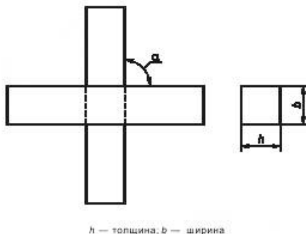
Рисунок 1 — Схема крестообразного образца
