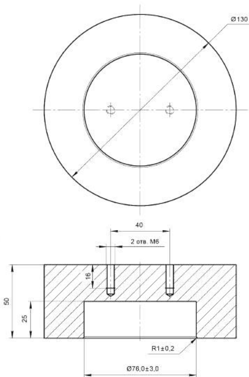
Рисунок ДБ.1 — Эскиз опорной наковальни
