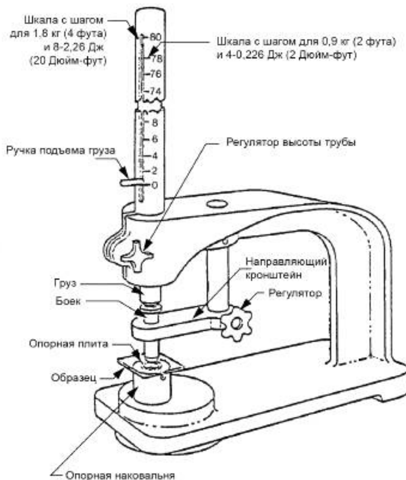
Рисунок ДД.1 — Установка для испытаний на удар
