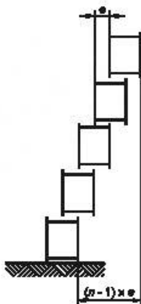
в) Смещение, приводящее к поперечным отклонениям
