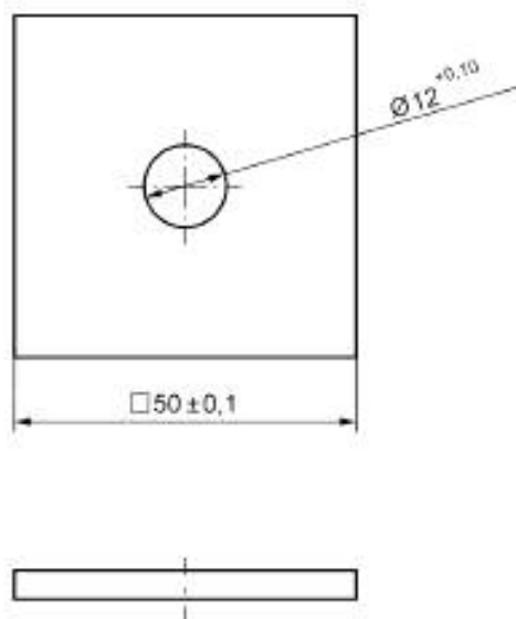
Рисунок 1 — Образец из ПК для испытаний на срез
