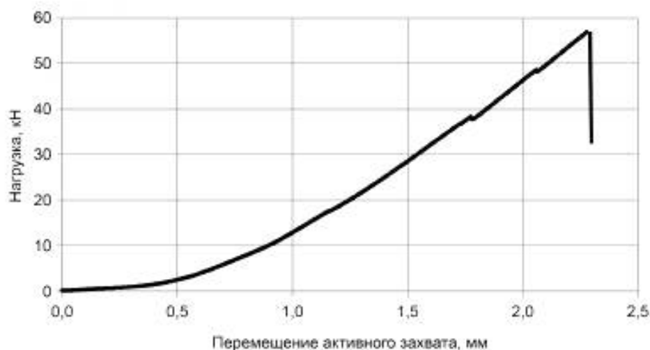
Рисунок 2 — Типовая диаграмма деформирования
