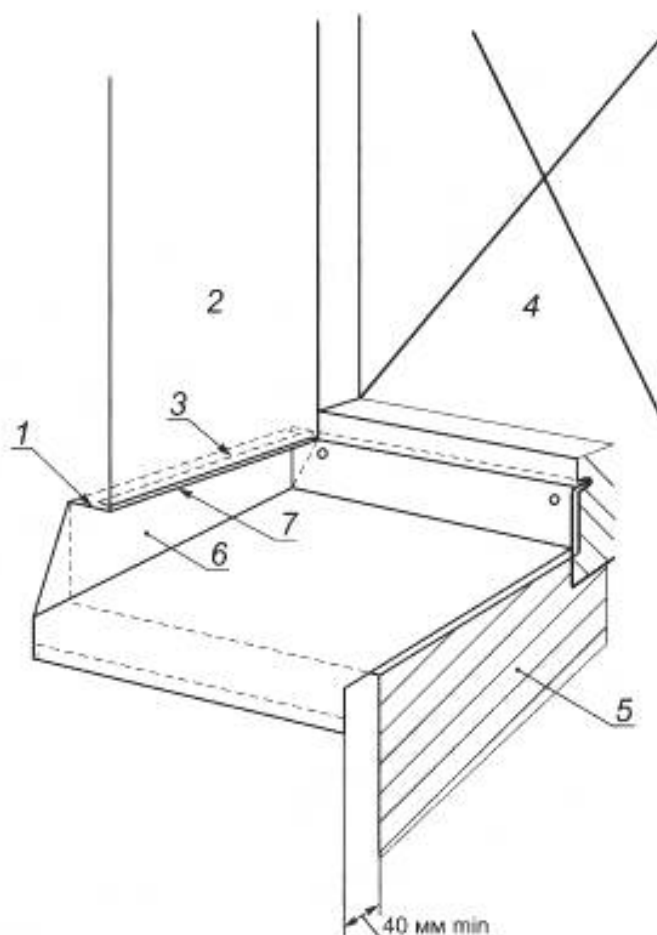
с) Подоконник из керамических пластин в два слоя
