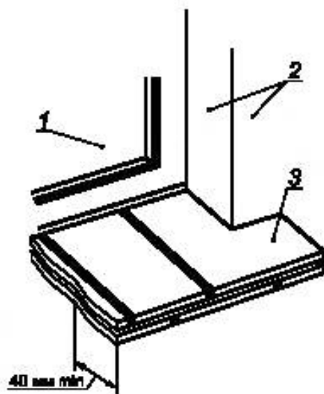
с) Подоконник из керамических пластин в два слоя
