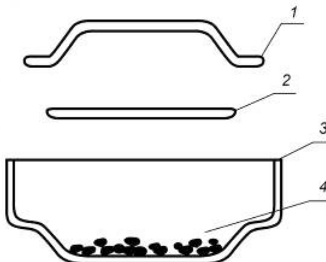
1 — герметичная крышка; 2 — диск 75 × 5,9 мм; 3 — герметичный тигель; 4 — образец
