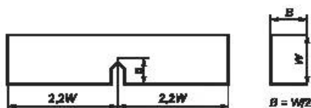
а — образец для трехточечного изгиба (SENB)
