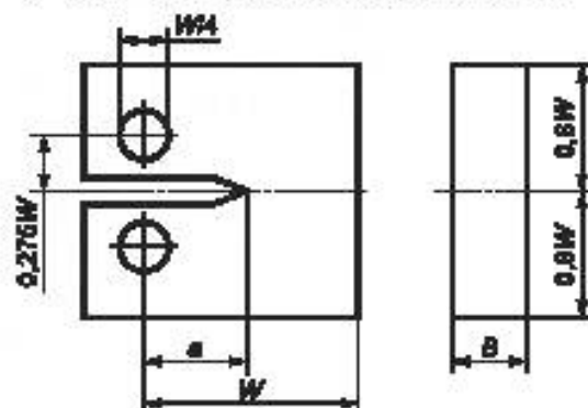
б — образец для централизованного растяжения (СТ)
