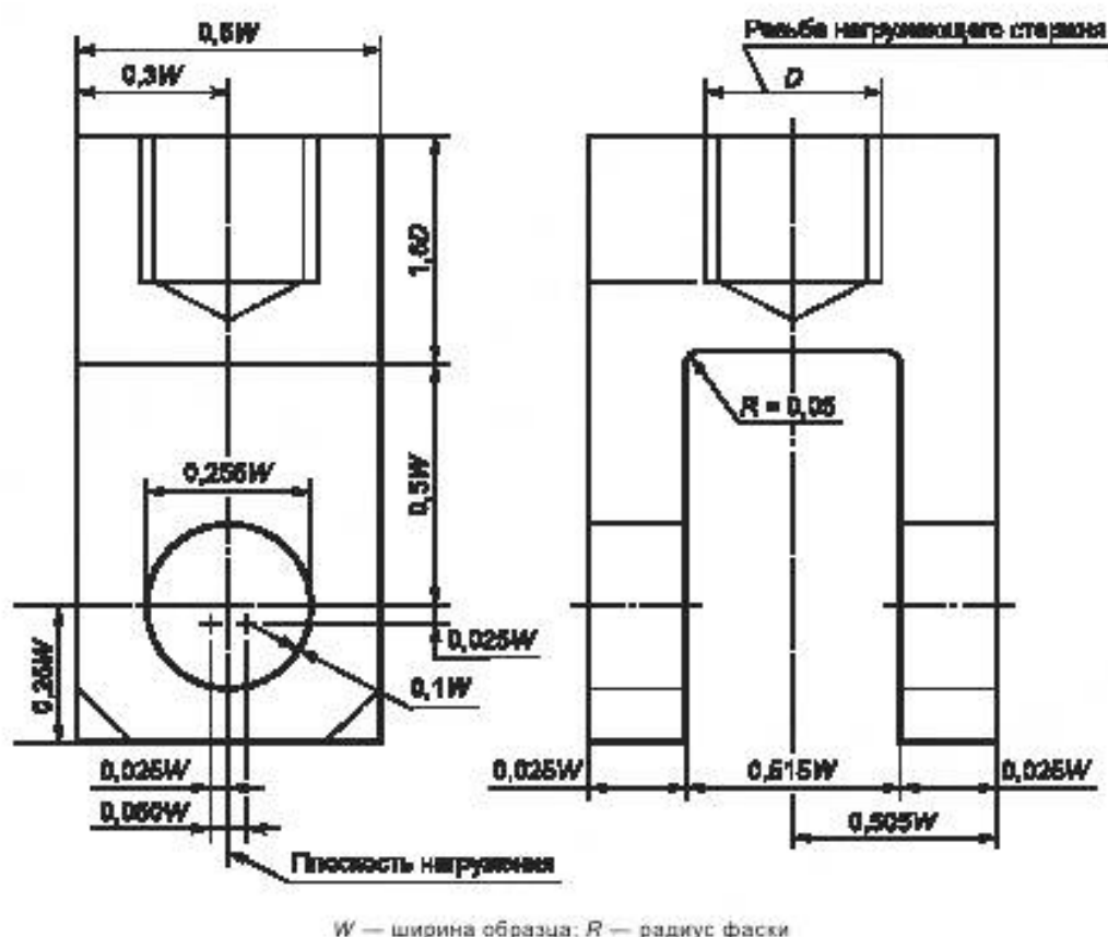
Рисунок 2 — Конструкция нагрузочной скобы для испытания на внецентренное растяжение для СТ
