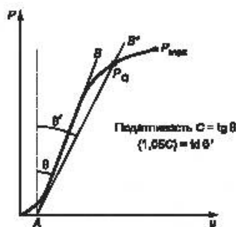
Рисунок 5 — Определение C и P_Q
