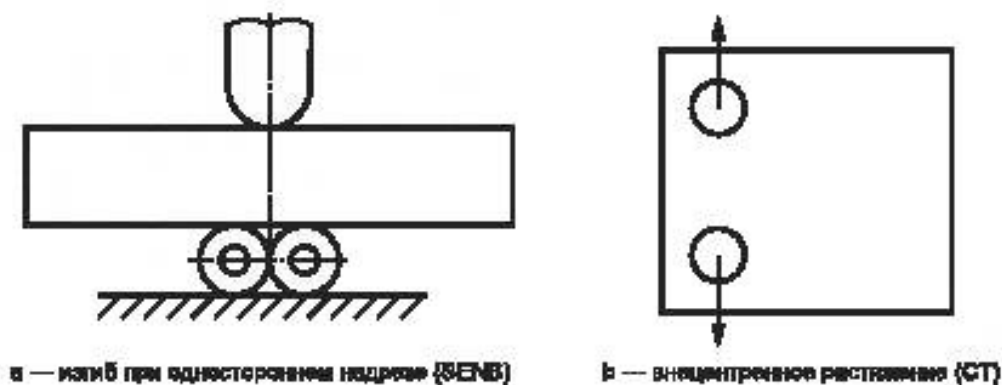
Рисунок 4 — Определение поправки смещения при вдавливании
