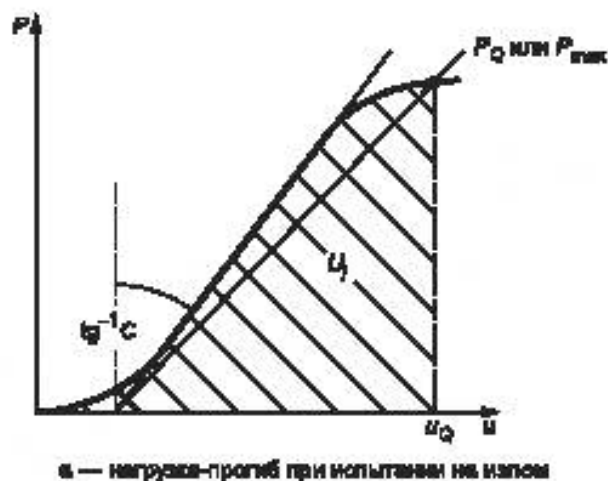
Рисунок 6. лист 1 — Метод поправки на вдавливание
