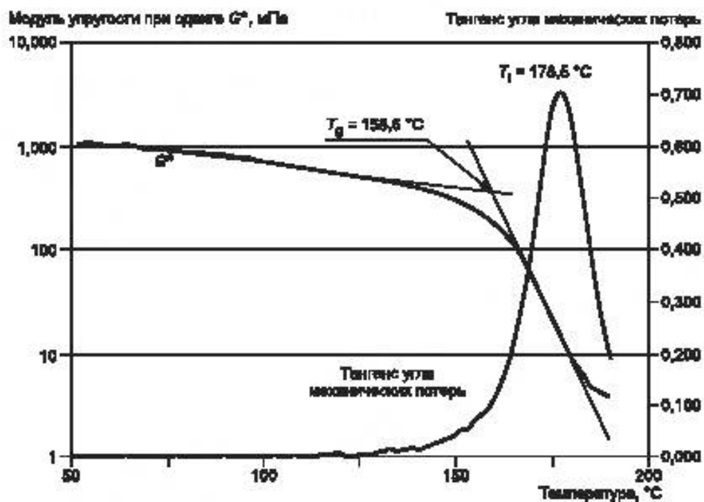
Рисунок 8 — Динамические методы определения температуры стеклования T_g после отверждения или T_1 линейным изменением температуры
