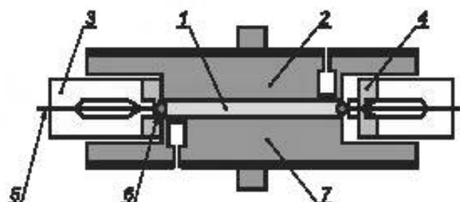
1 — образец; 2 — верхняя форма; 3 — пластины; 4 — уплотнение формы; 5 — разделительная пленка; 6 — уплотнительное кольцо; 7 — нижняя форма
