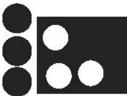
Рисунок 3 — Нарезка дисков из листа материала при помощи кольцевого вырубного штампа
