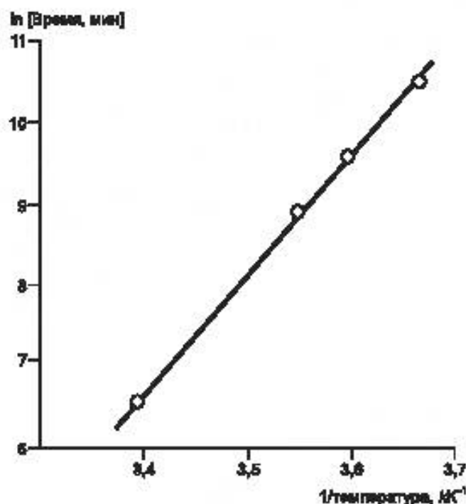
Рисунок 4 — График зависимости \ln[\Delta t] от 1/T
