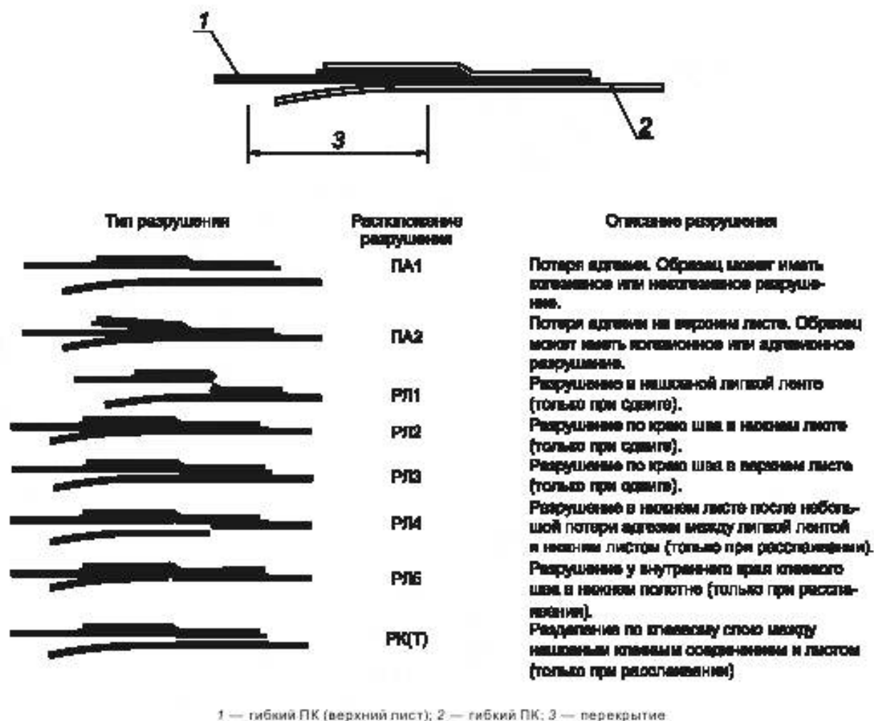
Рисунок 4 — Типы и расположения разрушений для образцов клеевого соединения внахлест, выполненного нашовным клеевым соединением
