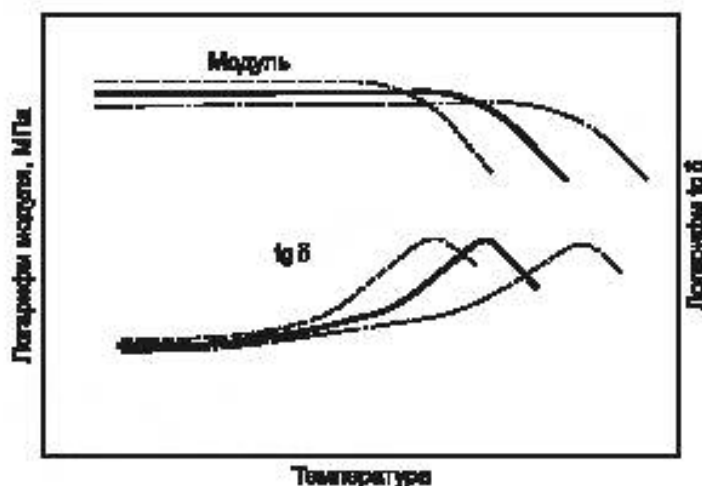
Рисунок 1 — Динамические механические свойства при сжатии (при различных частотах)
