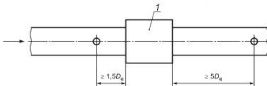
1 — вентилятор
