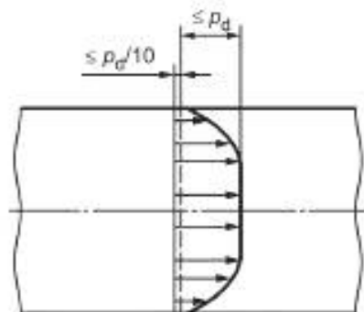
а) Идеальное распределение p_d
