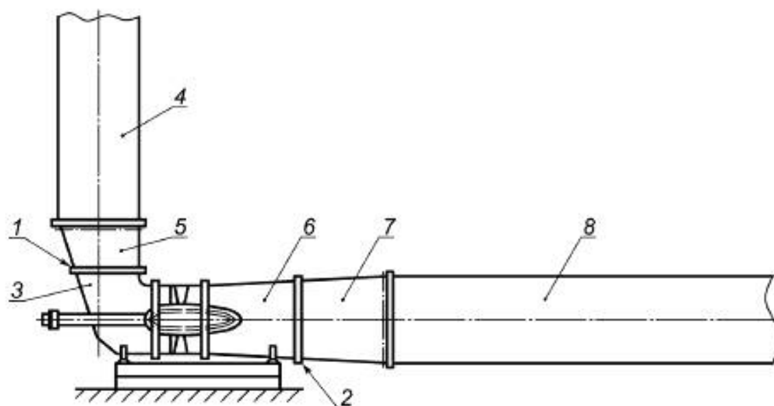
а) Осевой вентилятор
