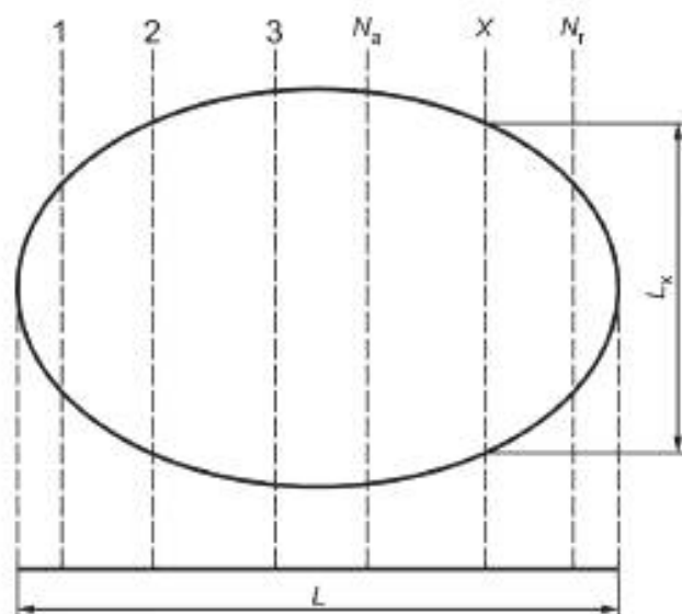
Рисунок 14 — Нормальное, но не прямоугольное или круглое сечение канала с примером распределения поперечных линий и точек измерения
