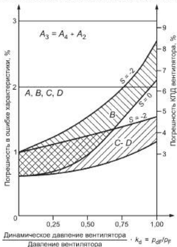
Рисунок 31 — Погрешность характеристики и погрешность КПД вентилятора
