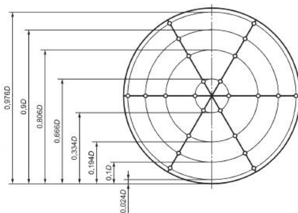
а) Распределение лог-Чебышева
