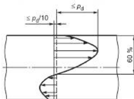
б) Хорошее распределение p_d
