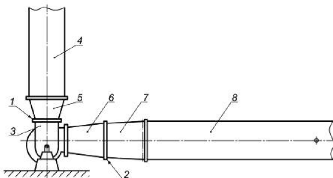
б) Радиальный вентилятор
