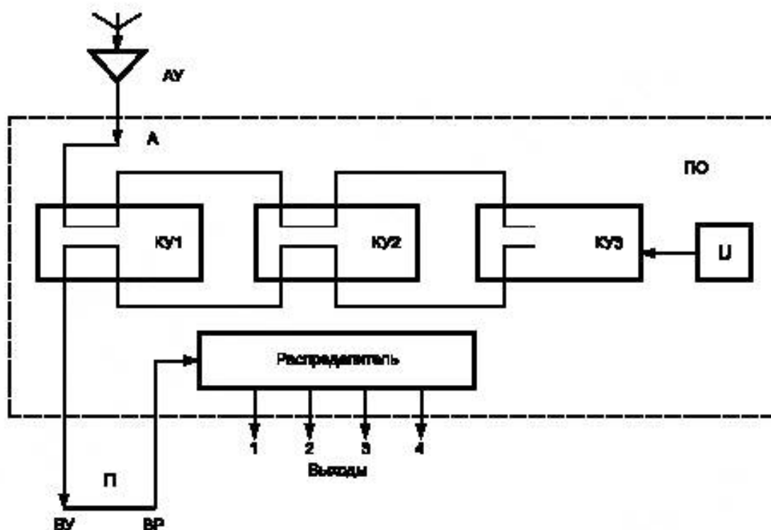
Рисунок А.3 — Приемное оборудование (ПО) системы коллективного приема
