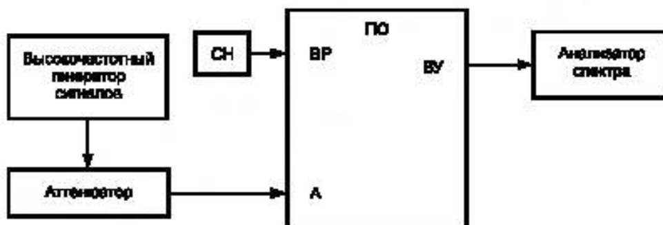
Рисунок 6 — Структурная схема для определения неравномерности АЧХ и избирательности ПО
