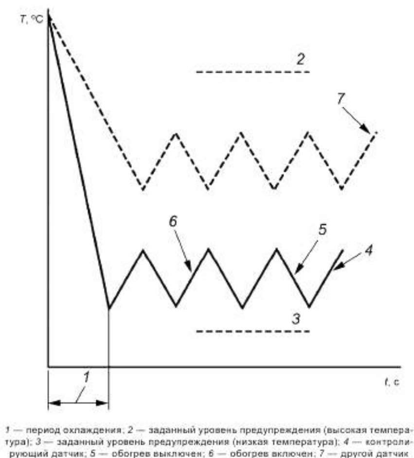
Рисунок D.1 — Типовая кривая регистрации времени обогрева
