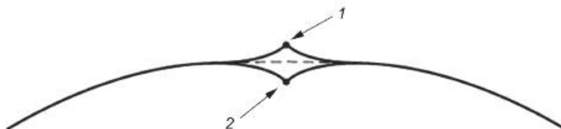
1 — наружная угловая деформация; 2 — внутренняя угловая деформация
