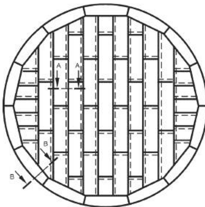
а) С кольцевыми окрайками по периметру
