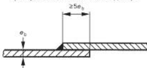
б) Разрез А-А, нахлест листов днища
