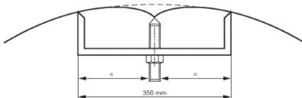
Рисунок 6 — Шаблон для измерения угловой деформации
