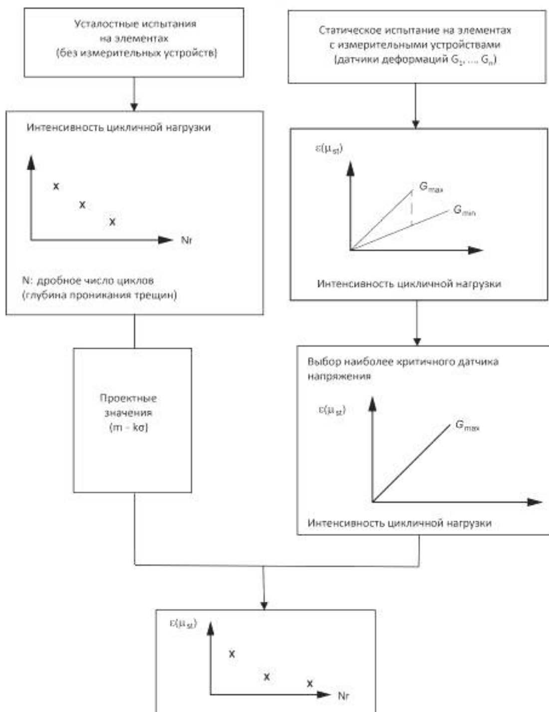
Рисунок В.1 — Блок-схема для мембран
