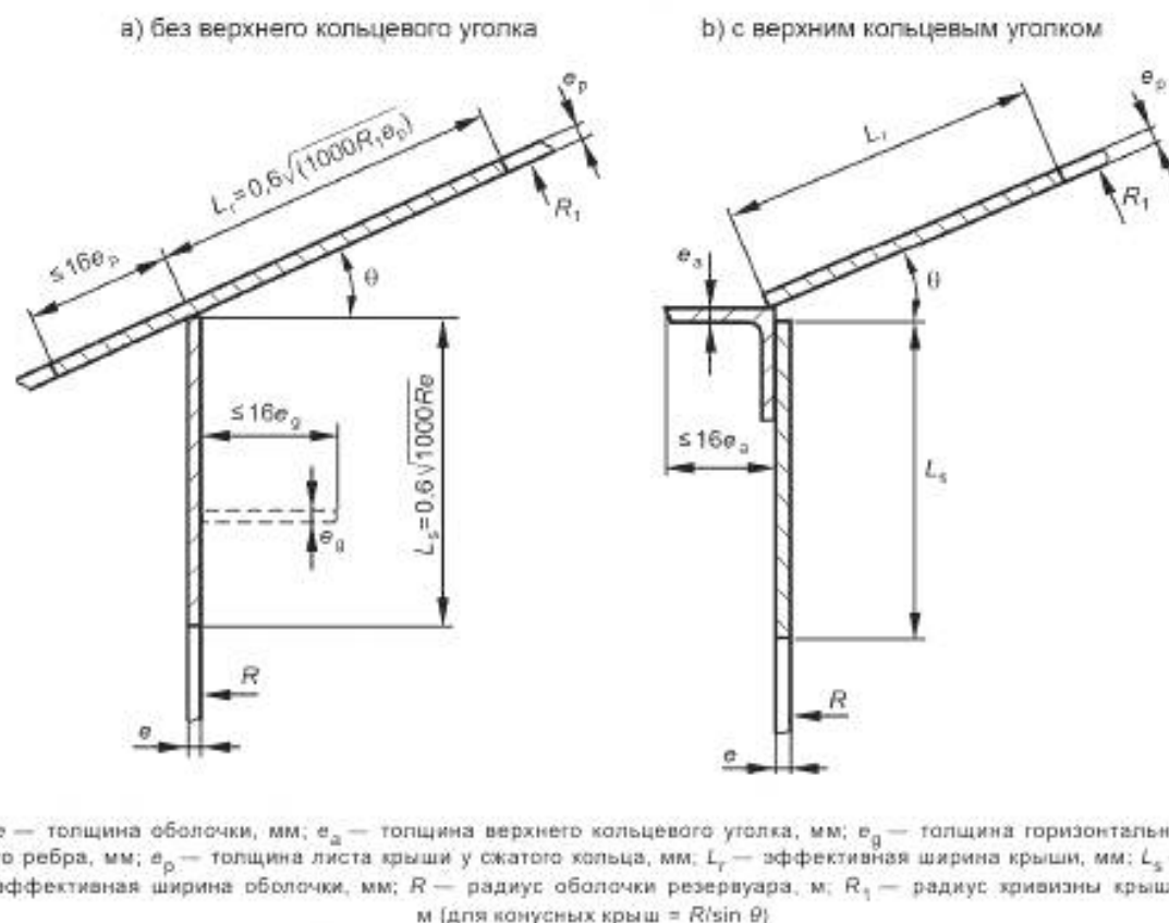
Рисунок 3 — Типовые зоны сжатия оболочки-крыши
