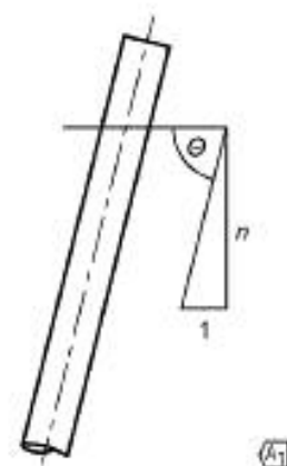
Рисунок 4 — Определение наклона сваи
