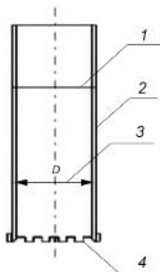
а) Обсадка трубами
