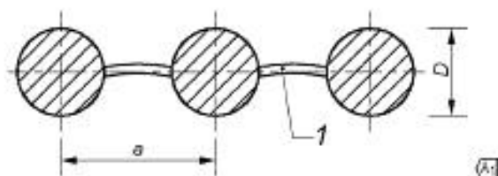
в) Буровые сваи, установленные с определенным шагом и объединенные между собой
