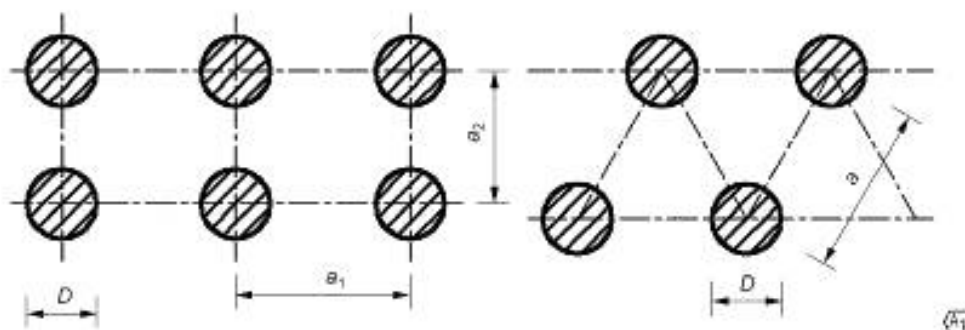
Рисунок 5 — Примеры группы свай
