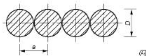
б) Баррета из бурокасательных свай
