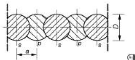
а) Баррета из буросекущих свай
