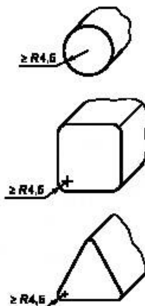
Рисунок 4 — Закругления деталей
