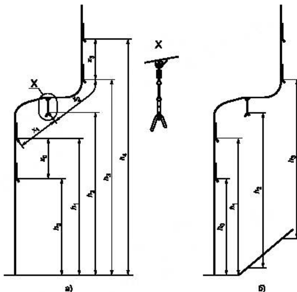
Рисунок 2 — Схема и расположение постоянных оттяжек
