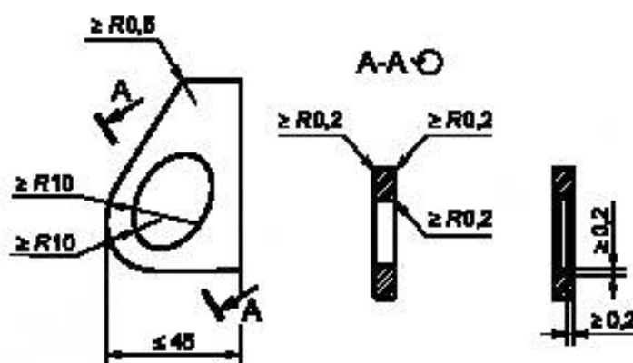
Рисунок 3 — Исполнение индивидуальных точек страховки
