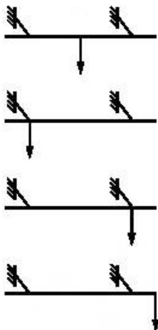
Рисунок E.3 — Схема испытательных нагрузок для коллективных верхних систем страховки
