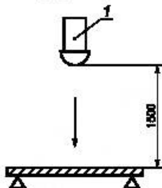
б) Вертикальный удар по горизонтальной поверхности
