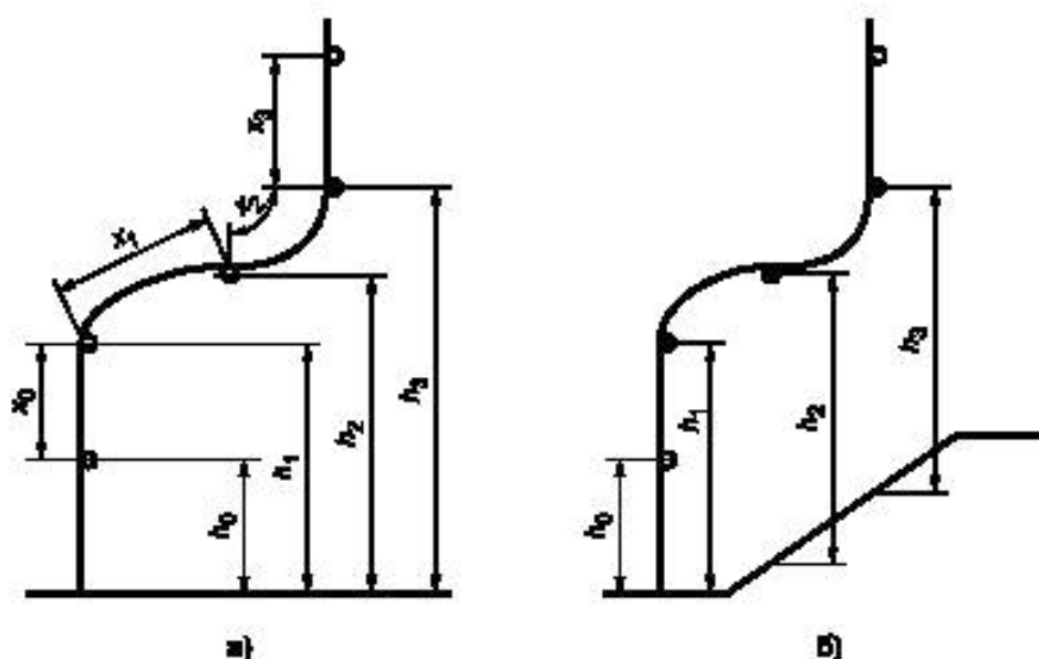
Рисунок 1 — Расположение точек страховки
