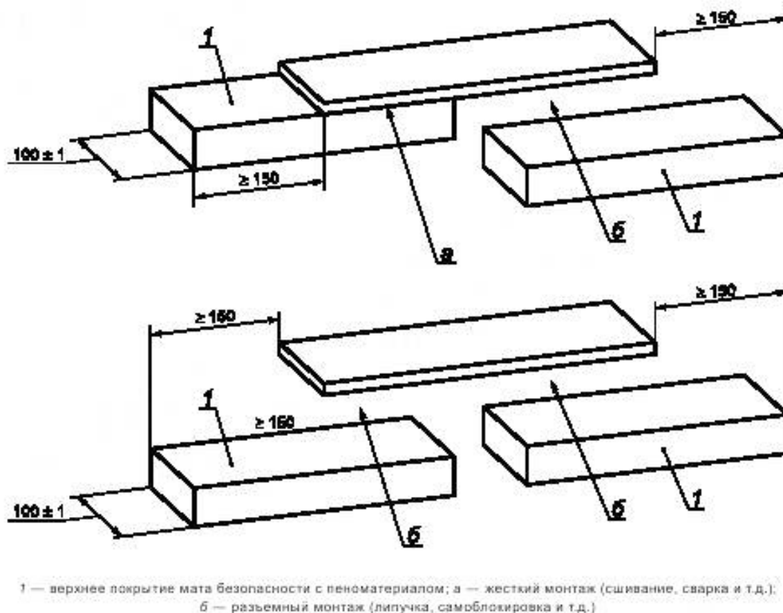
Рисунок Ж.1 — Пример соединений
