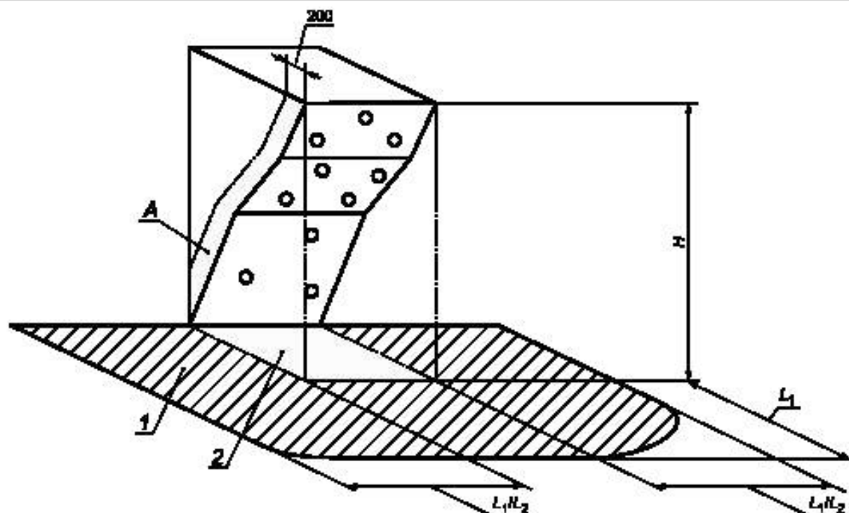
1 — верхняя поверхность области удара; 2 — проекция стены для боулдеринга; H — высота наиболее высокого возможного зацепа; L_1 — дополнительная длина, добавляемая к проекции стены для боулдеринга спереди; L_2 — дополнительная ширина области удара (при особых условиях); А — боковые поверхности, по которым возможно передвижение (рассматриваются как часть передней стены)
