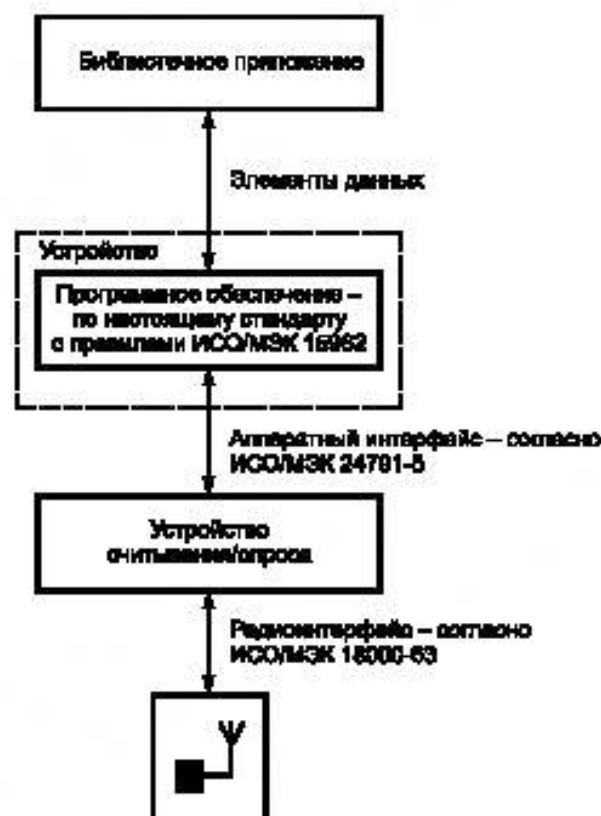
Рисунок 2 — Архитектура с интегрированными программными компонентами
