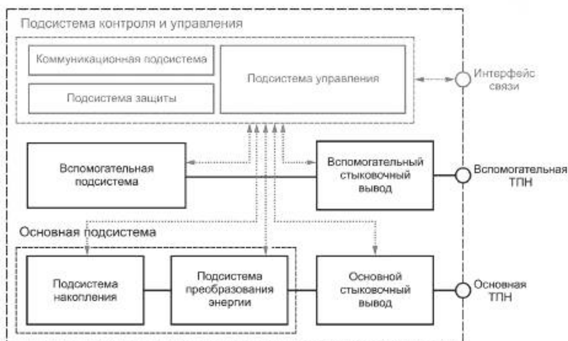
Рисунок 8 — Архитектура СНЭЭ в двух основных конфигурациях, лист 1
