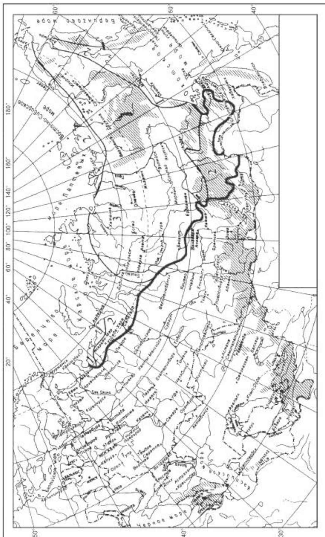
Схематическая карта северной строительно-климатической зоны
