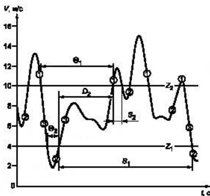
Рисунок Б.1 — Определение длительностей штормов ( S ), окон погоды ( \Theta ) и продолжительностей ситуаций в интервале ( D )
