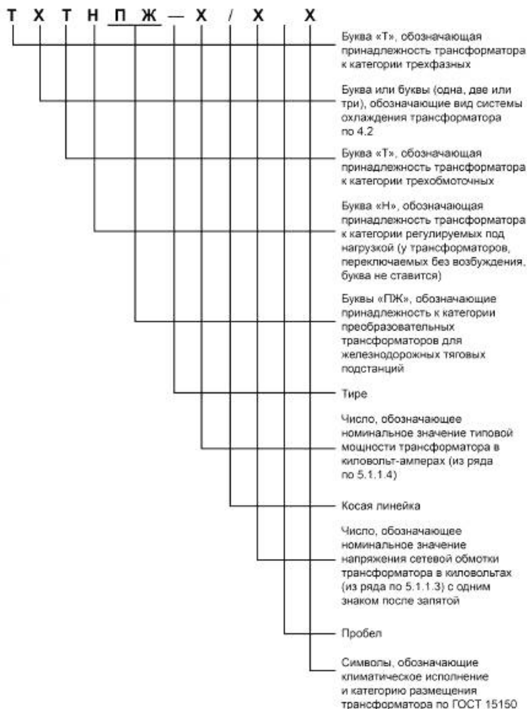
Рисунок 1 — Структурная схема условного обозначения трансформатора
