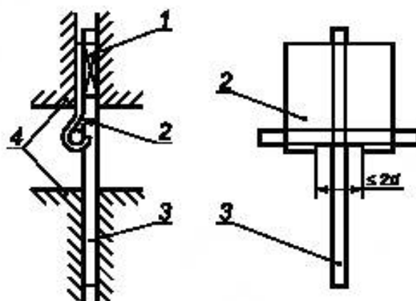
1 — вкладыш; 2 — крючкообразный натяжитель; 3 — испытуемый образец; 4 — зажимные кулачки натяжного устройства; d — диаметр проволоки
