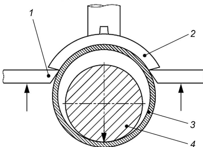
1 — зажимное устройство; 2 — седловой отвод из ПЭ; 3 — труба из ПЭ; 4 — нагружающий стержень
