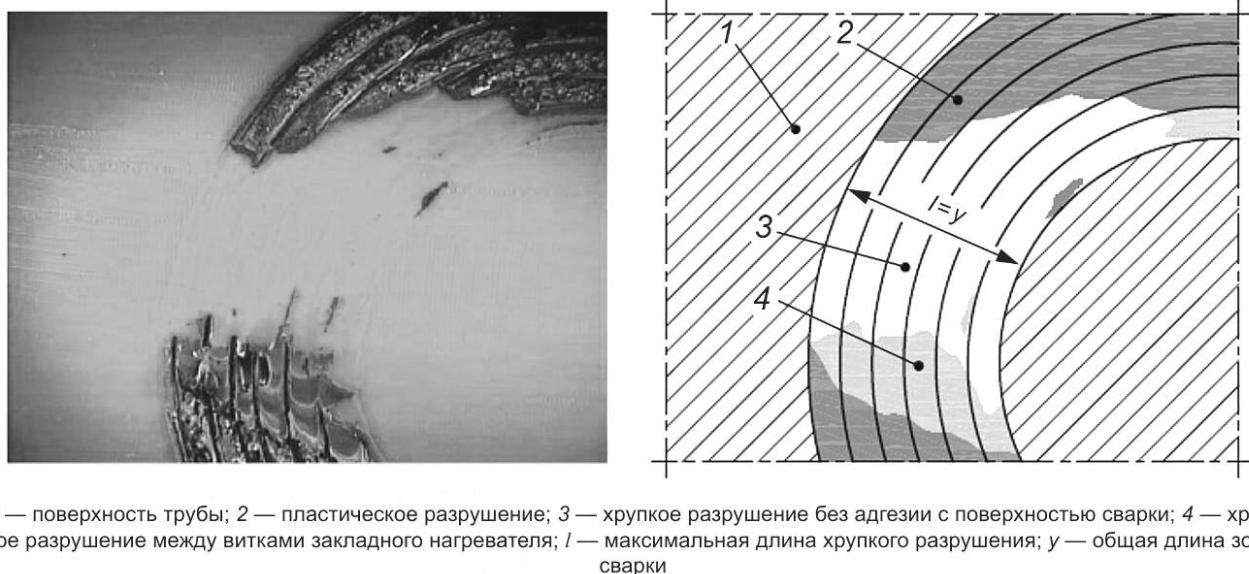
Рисунок ДБ.5 — Пример хрупкого разрушения на поверхности сварки
