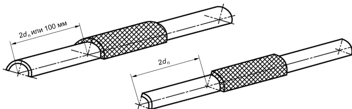
Рисунок ДА.1 — Подготовка испытываемых образцов
