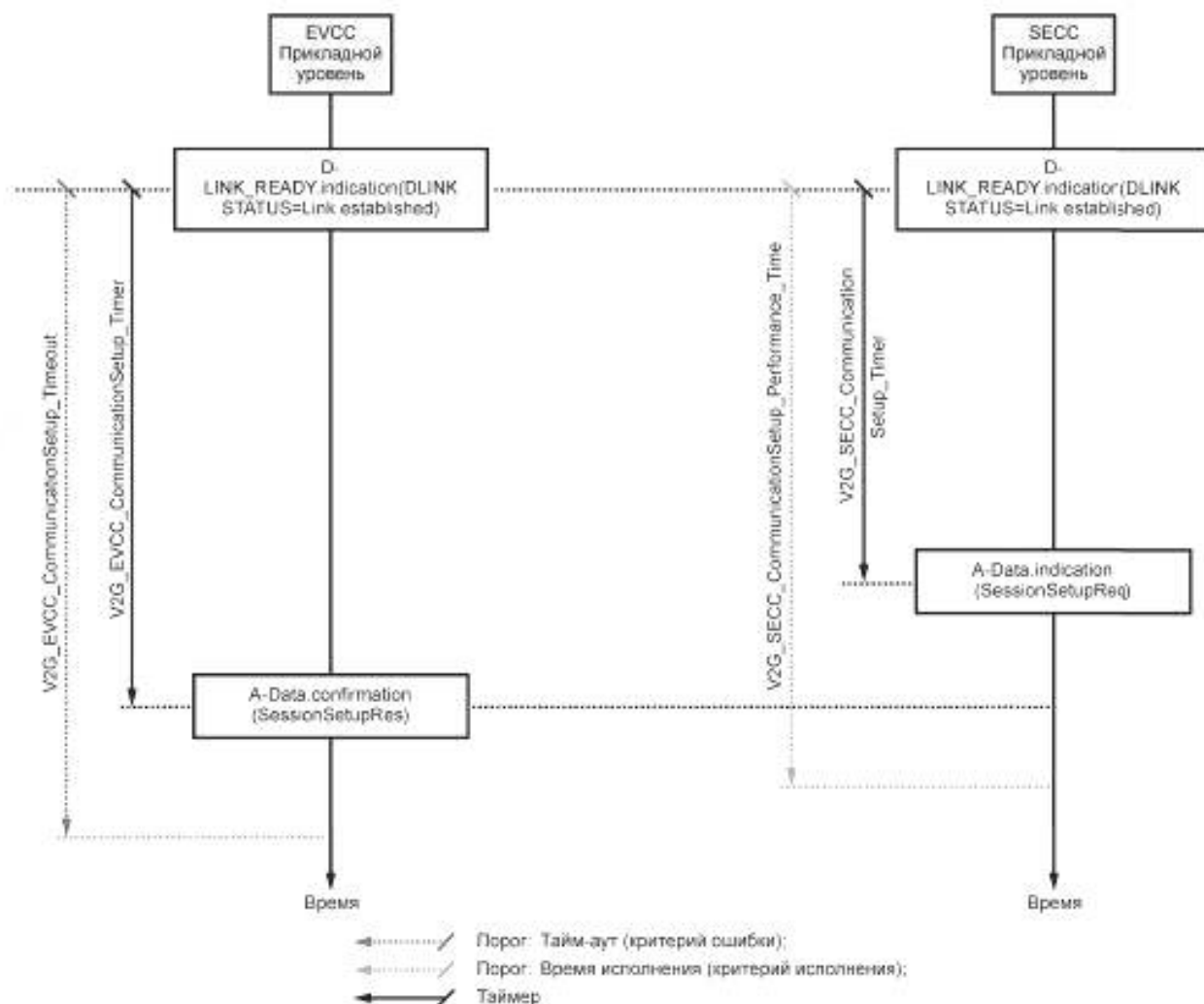
Рисунок 99 — Хронирование установления связи
