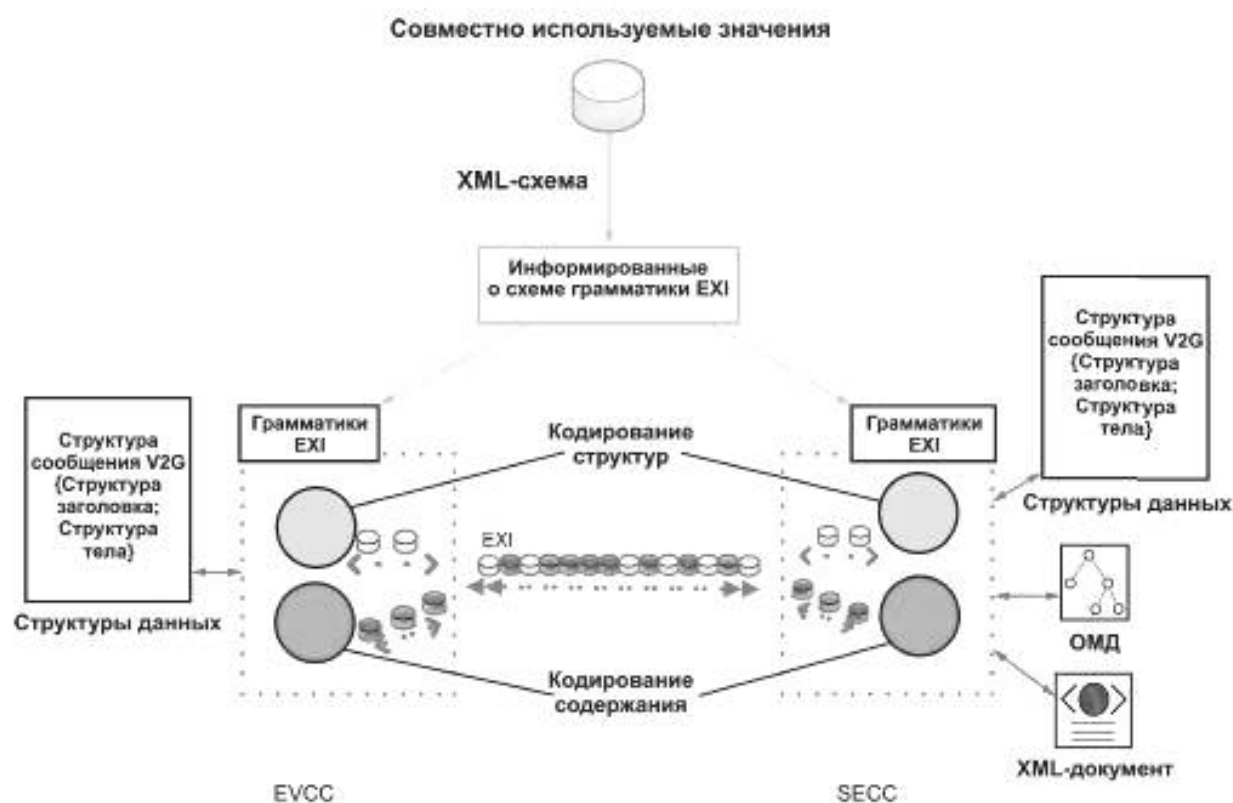
Рисунок 11 — Применение базовой концепции EXI к связи V2G
