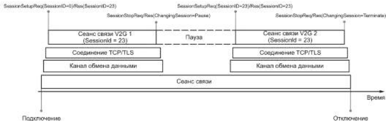
Рисунок 22 — Обработка сеанса связи V2G
