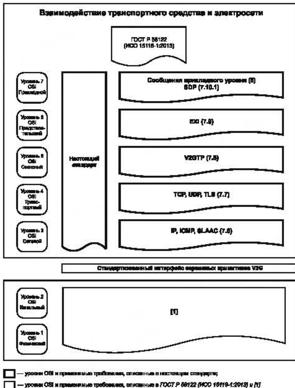
Рисунок 2 — Обзор связи документов V2G
