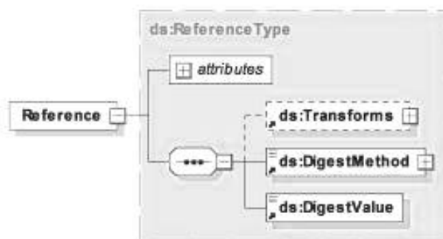
Рисунок 13 — Диаграмма — Элемент Reference, включенный в элемент SignedInfo
