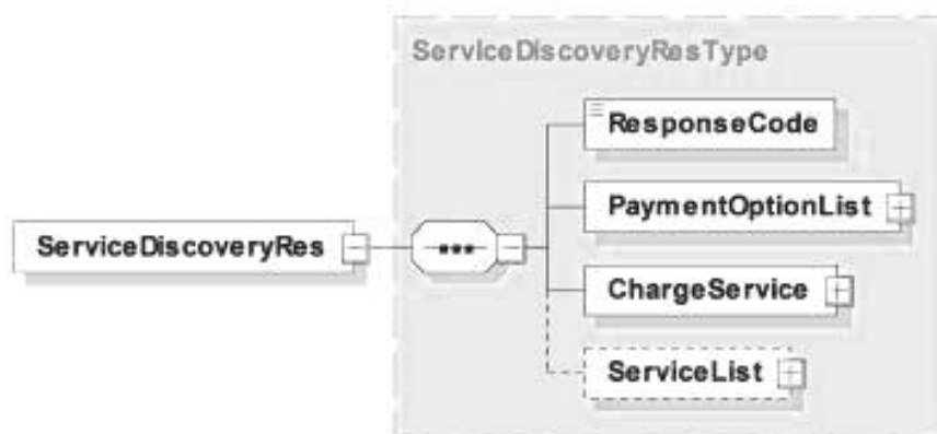
Рисунок 26 — Диаграмма — ServiceDiscoveryRes
