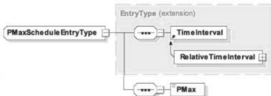
Рисунок 71 — Диаграмма — PMaxScheduleEntryType
