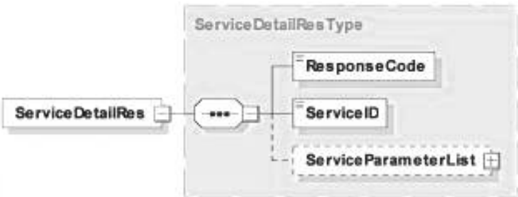
Рисунок 28 — Диаграмма — ServiceDetailRes
