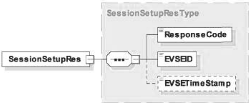
Рисунок 24 — Диаграмма — SessionSetupRes
