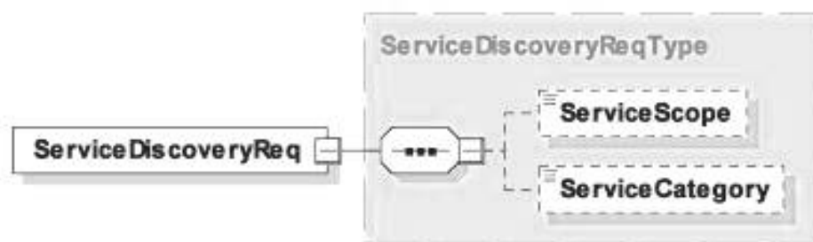
Рисунок 25 — Диаграмма — ServiceDiscoveryReq
