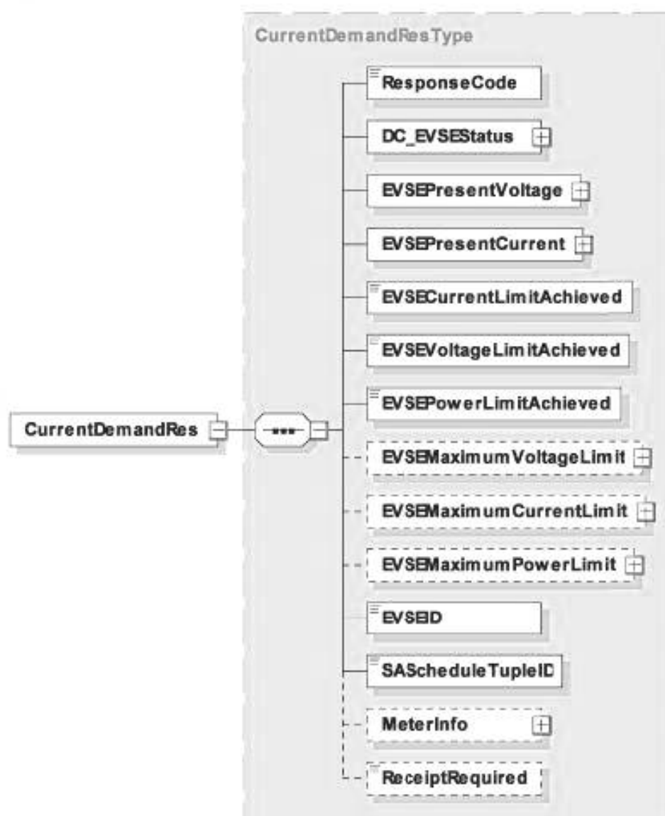
Рисунок 54 — Диаграмма — CurrentDemandRes
