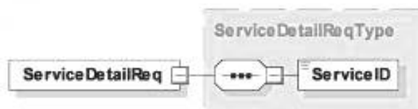
Рисунок 27 — Диаграмма — ServiceDetailReq
