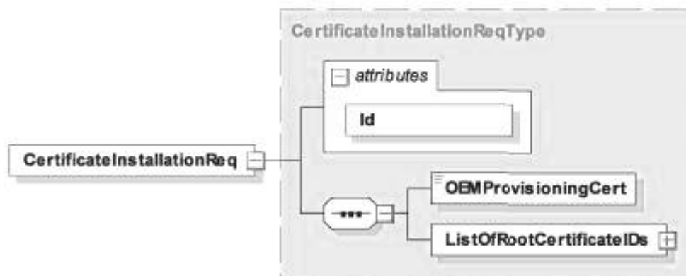
Рисунок 41 — Диаграмма — CertificateInstallationReq
