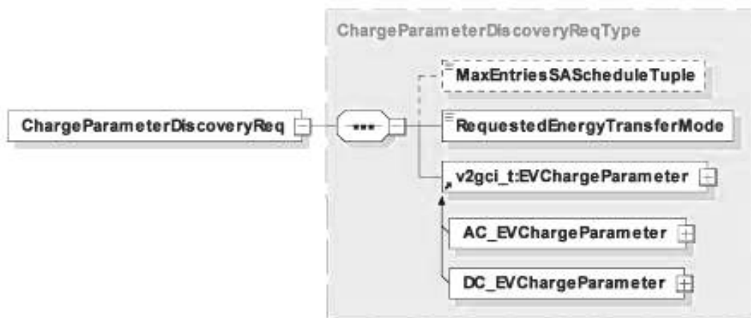
Рисунок 35 — Диаграмма — ChargeParameterDiscoveryReq
