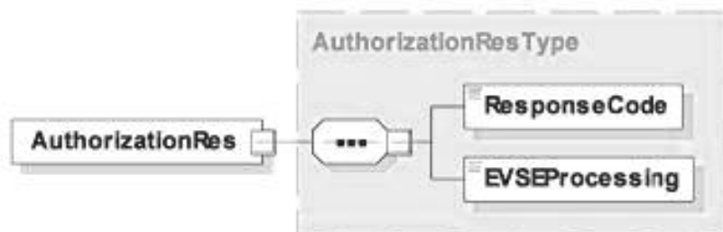
Рисунок 34 — Диаграмма — AuthorizationRes
