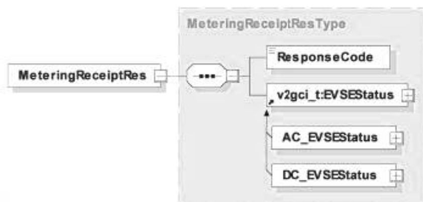
Рисунок 46 — Диаграмма — MeteringReceiptRes
