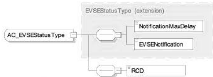
Рисунок 87 — Диаграмма — AC_EVSEStatusType
