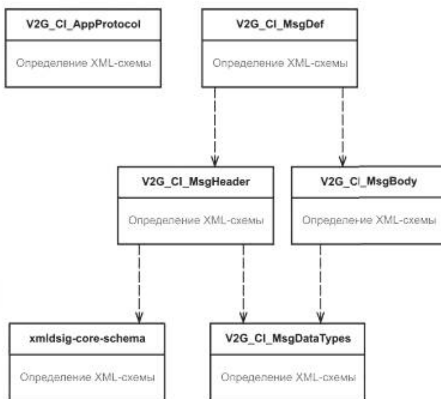
Рисунок F.1 — Диаграмма зависимости определений XML-схемы V2G
