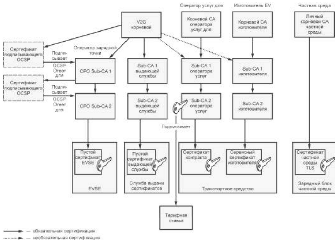
Рисунок С.1 — Обзор структуры сертификатов
