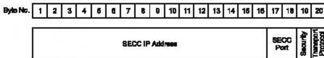
Рисунок 16 — Полезные данные сообщения об обнаружении SECC
