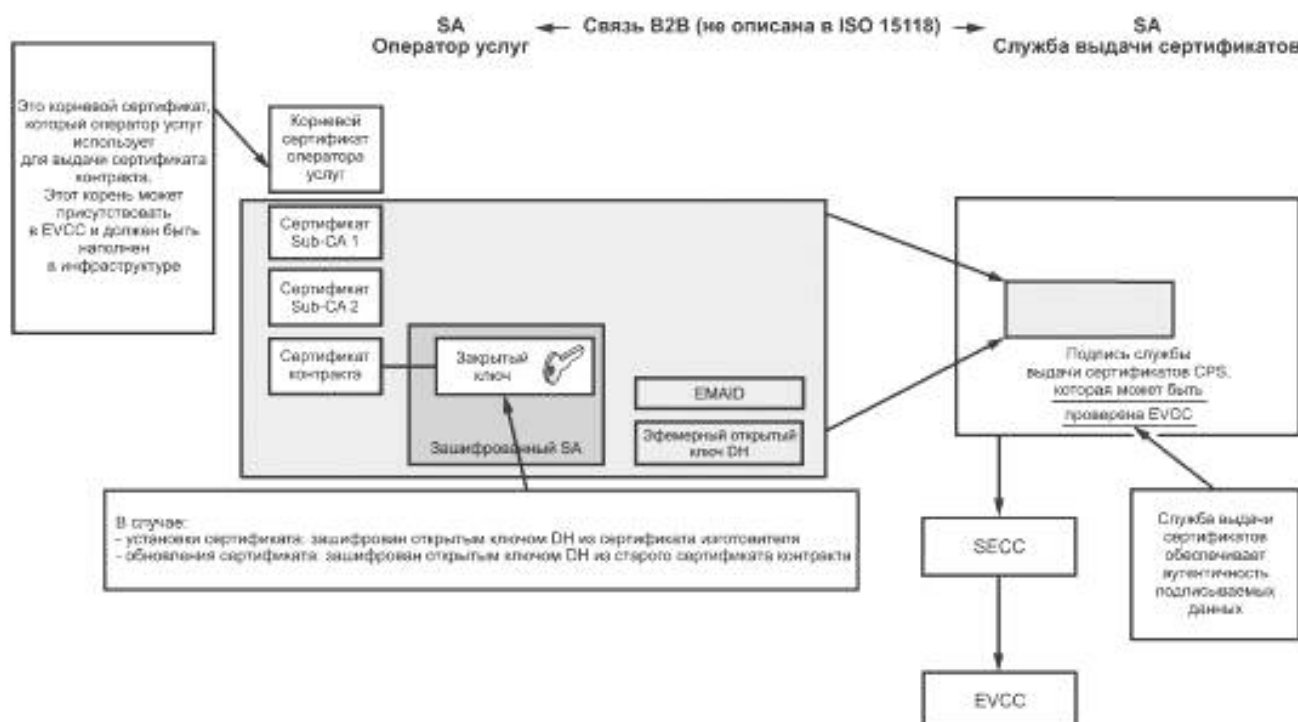
Рисунок 14 — Процесс для CertificateInstallationRes и CertificateUpdateRes
