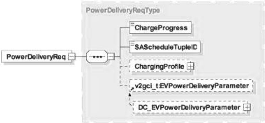
Рисунок 37 — Диаграмма — PowerDeliveryReq
