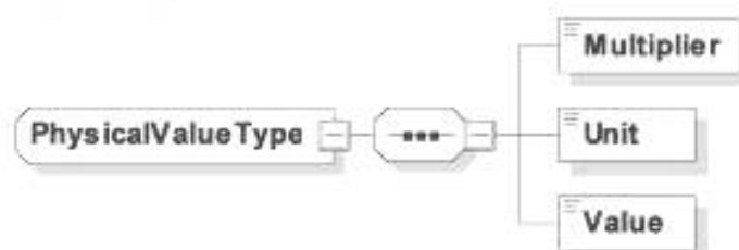
Рисунок 63 — Диаграмма — PhysicalValueType
