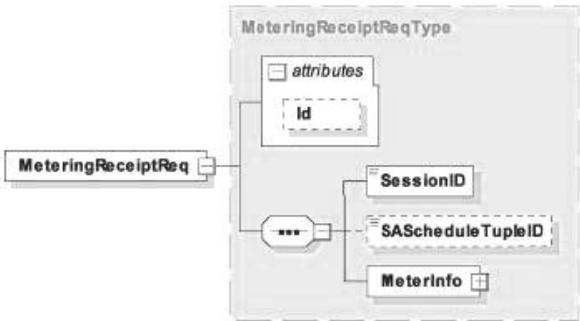
Рисунок 45 — Диаграмма — MeteringReceiptReq
