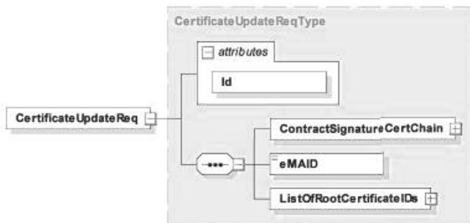
Рисунок 39 — Диаграмма — CertificateUpdateReq
