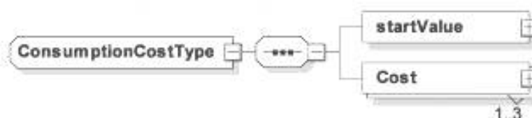
Рисунок 75 — Диаграмма — ConsumptionCostType
