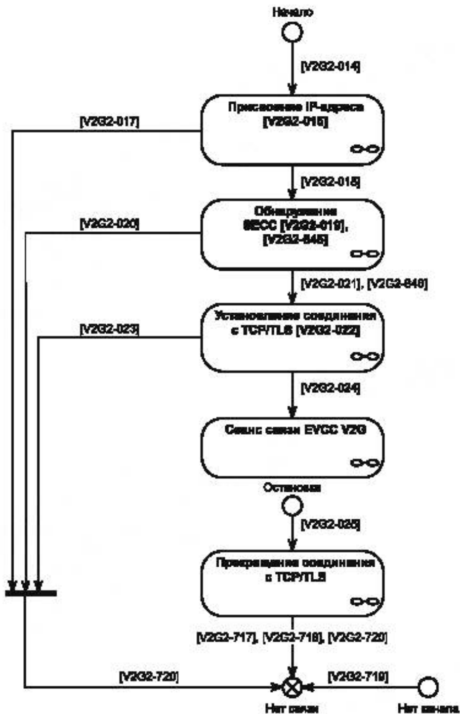
Рисунок 6 — Обзор коммуникационных состояний EVCC
