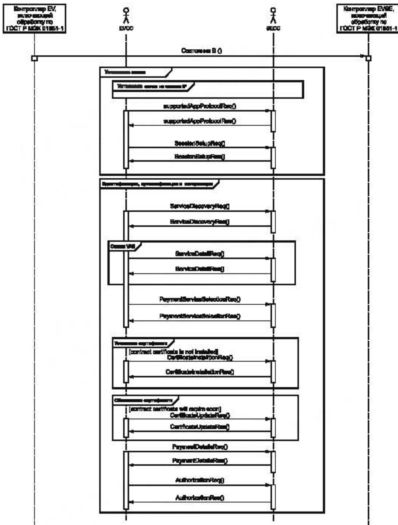
Рисунок 106 — Обзор последовательности сообщений запрос-ответ для переменного тока, идентификационный режим PnC (1 из 2)
