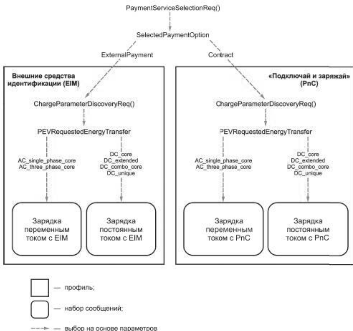
Рисунок 97 — Выбор наборов сообщений
