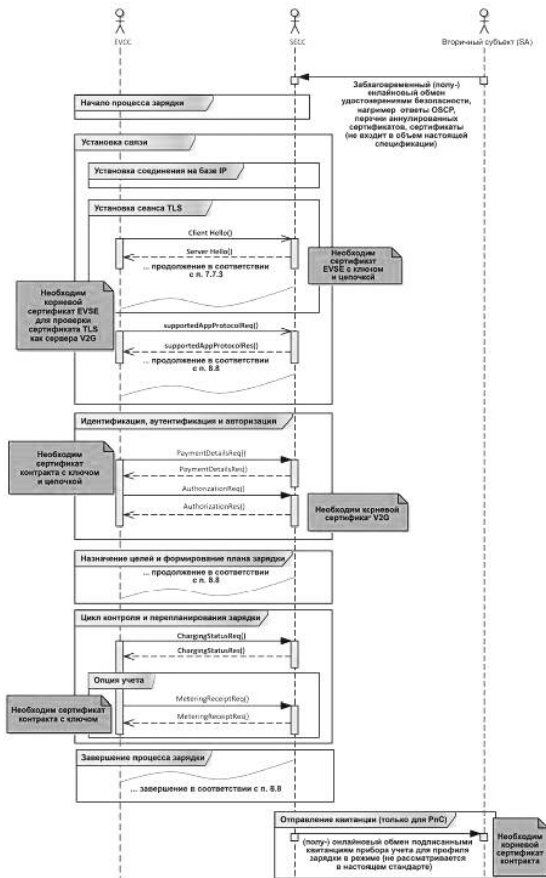
Рисунок 4 — Пример связи в полуонлайновом режиме
