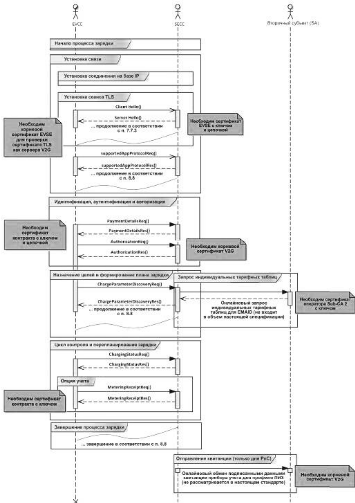
Рисунок 5 — Пример связи в онлайн-режиме
