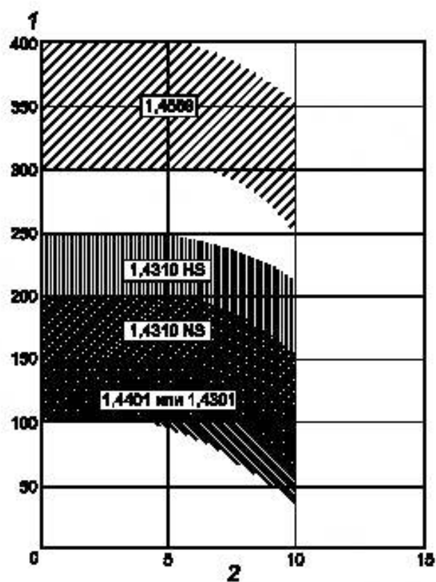
Рисунок А.1 — Повышение временного сопротивления холоднотянутой проволоки в результате термической обработки в соответствии с таблицей А.2
