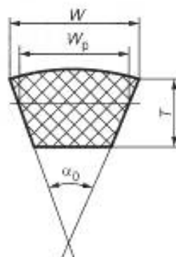
W — ширина большего основания, мм; W_p — расчетная ширина ремня, мм; T — высота ремня, мм; \alpha_0 — угол клина сечения ремня, град
