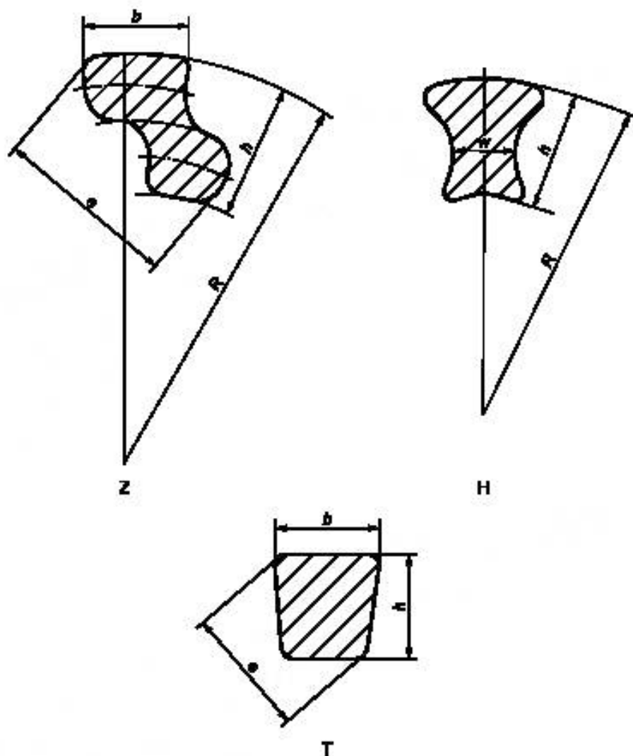
Рисунок 1 — Формы поперечных сечений фасонной проволоки
