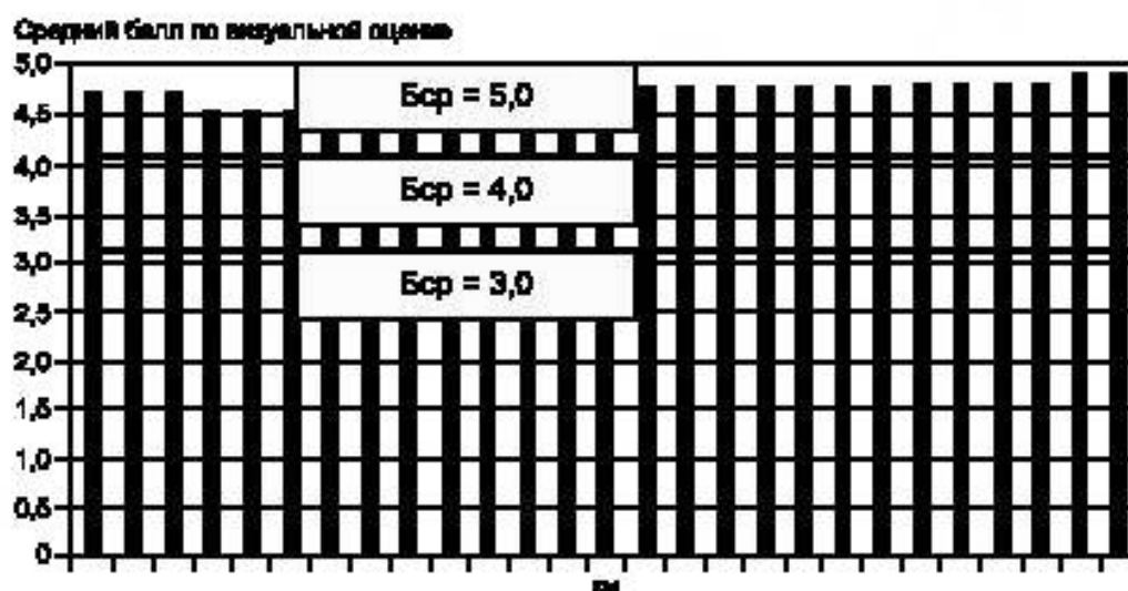
Рисунок А.4 — Средний балл по визуальной оценке (обратное направление)
