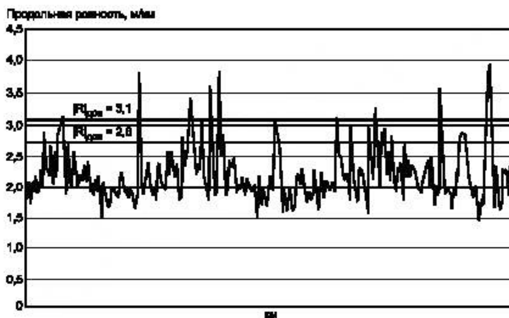
Рисунок А.5 — Продольная ровность покрытия нежесткой дорожной одежды, замеренная на участке по внешней полосе движения в прямом направлении (полоса 1)
