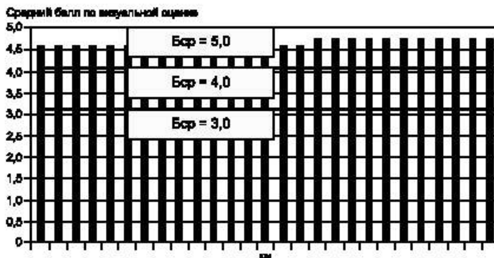
Рисунок А.3 — Средний балл по визуальной оценке (прямое направление)
