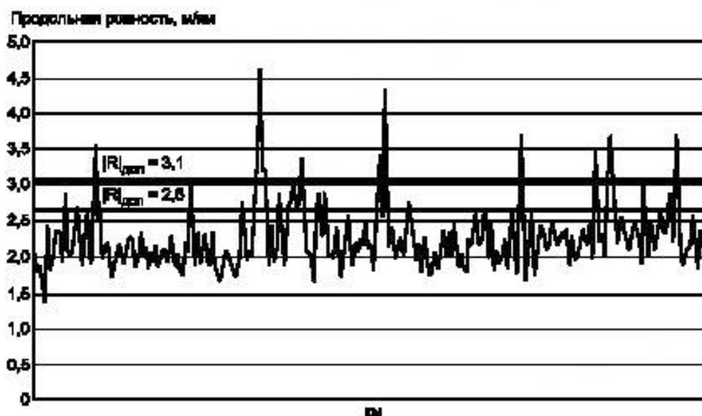
Рисунок А.6 — Продольная ровность покрытия нежесткой дорожной одежды, замеренная на участке по внутренней полосе движения в обратном направлении (полоса 4)
