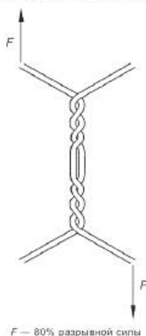
Рисунок 4 — Нагрузка на сетку для проверки прочности свивки
