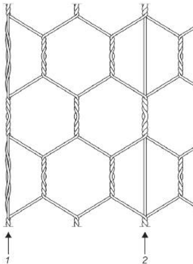
1 — бортовая проволока; 2 — проволочная растяжка
