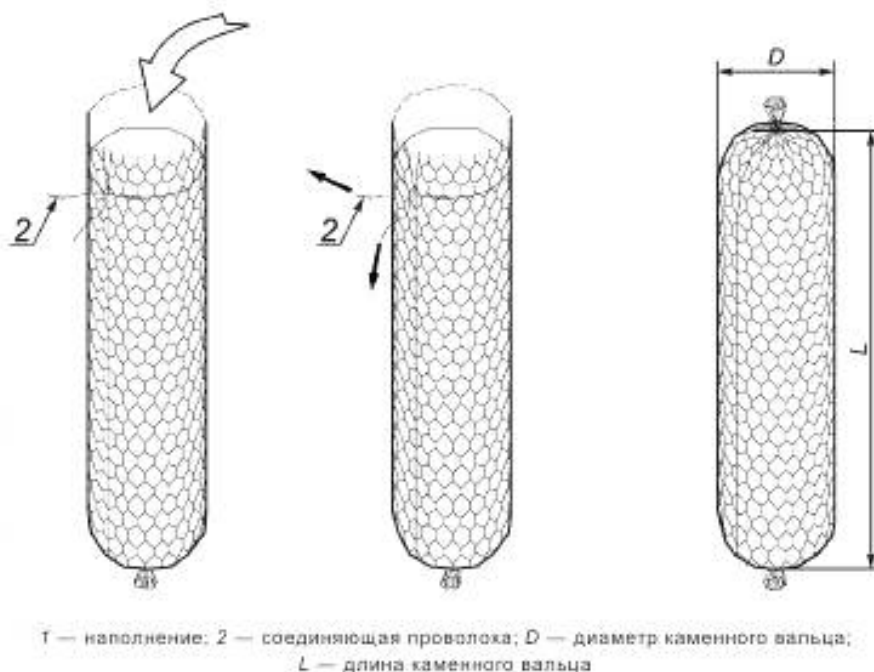
Рисунок 5 — Примеры каменных вальцов
