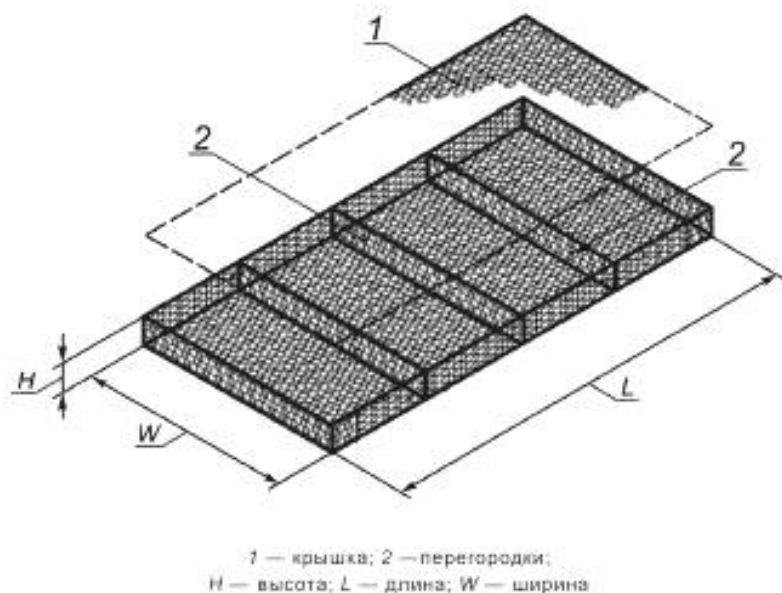
Рисунок 4 — Речной матрац
