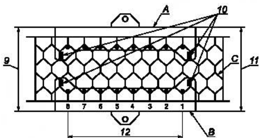
Рисунок 12 — Стыковочные металлические листы для проволоочной сетки типа 6 × 8
