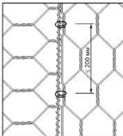
Рисунок 7 — С-образные кольца
