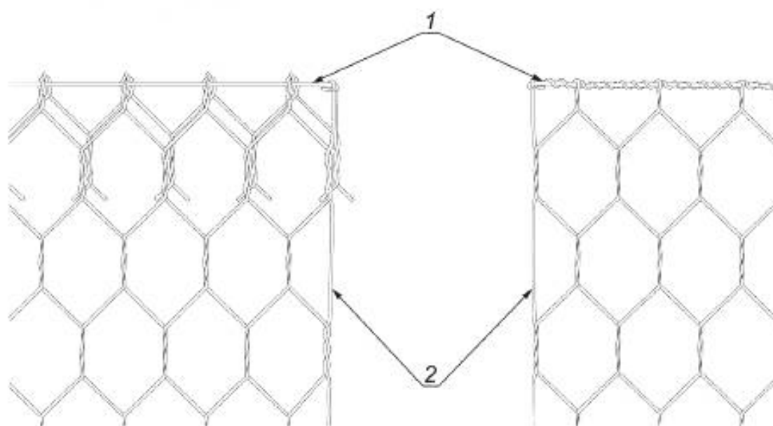
1 — продольная бортовая проволока; 2 — поперечная бортовая проволока
