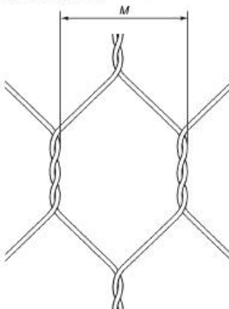
Рисунок 1 — Размер ячеек
