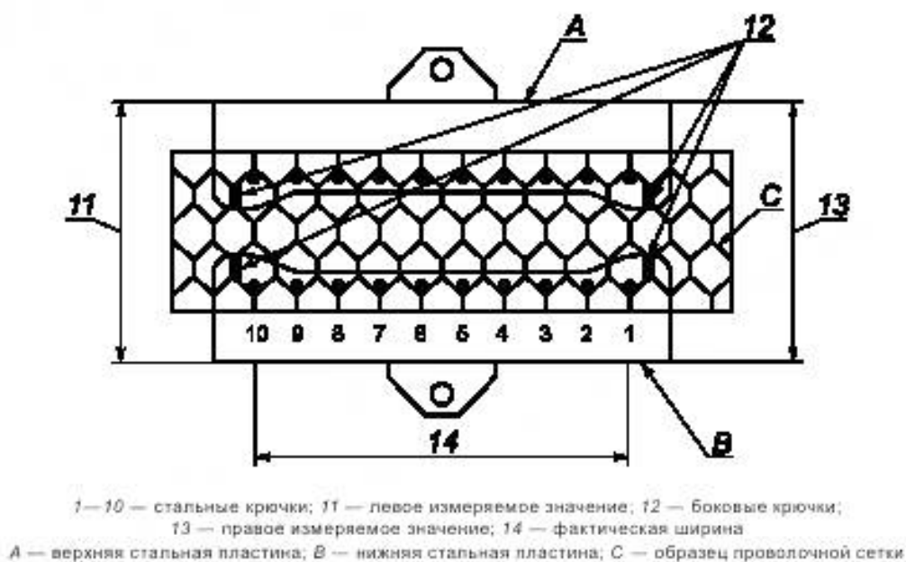
Рисунок 11 — Стыковочные металлические листы для проволоочной сетки типа 5 × 7
