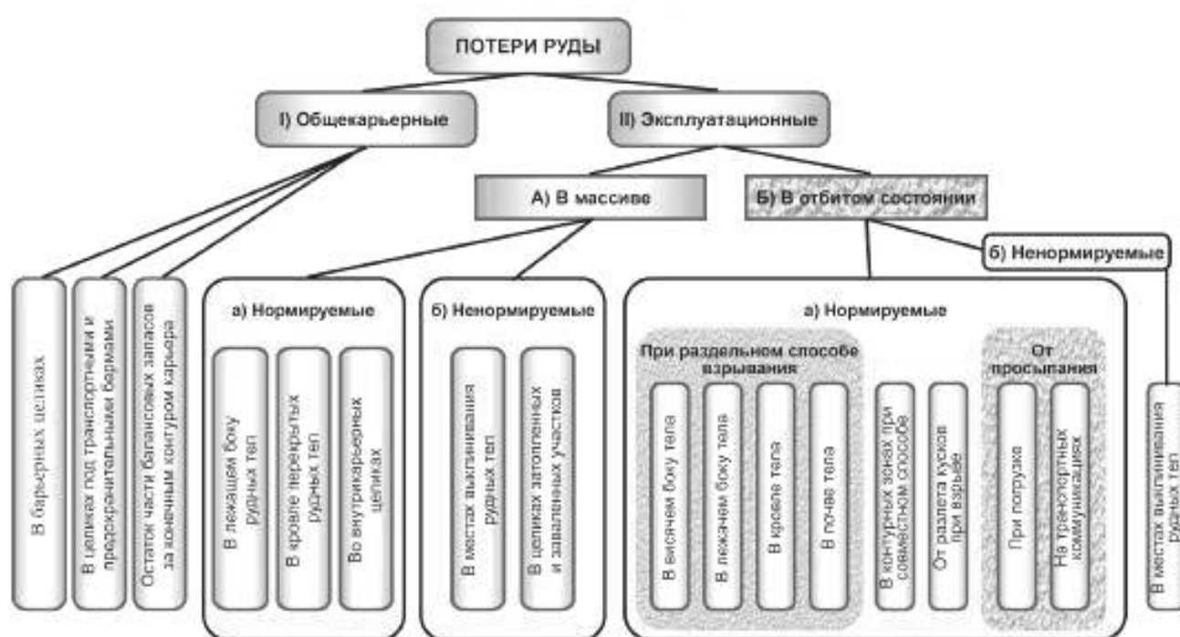
Рисунок 1 — Структура потерь алмазосодержащих руд
