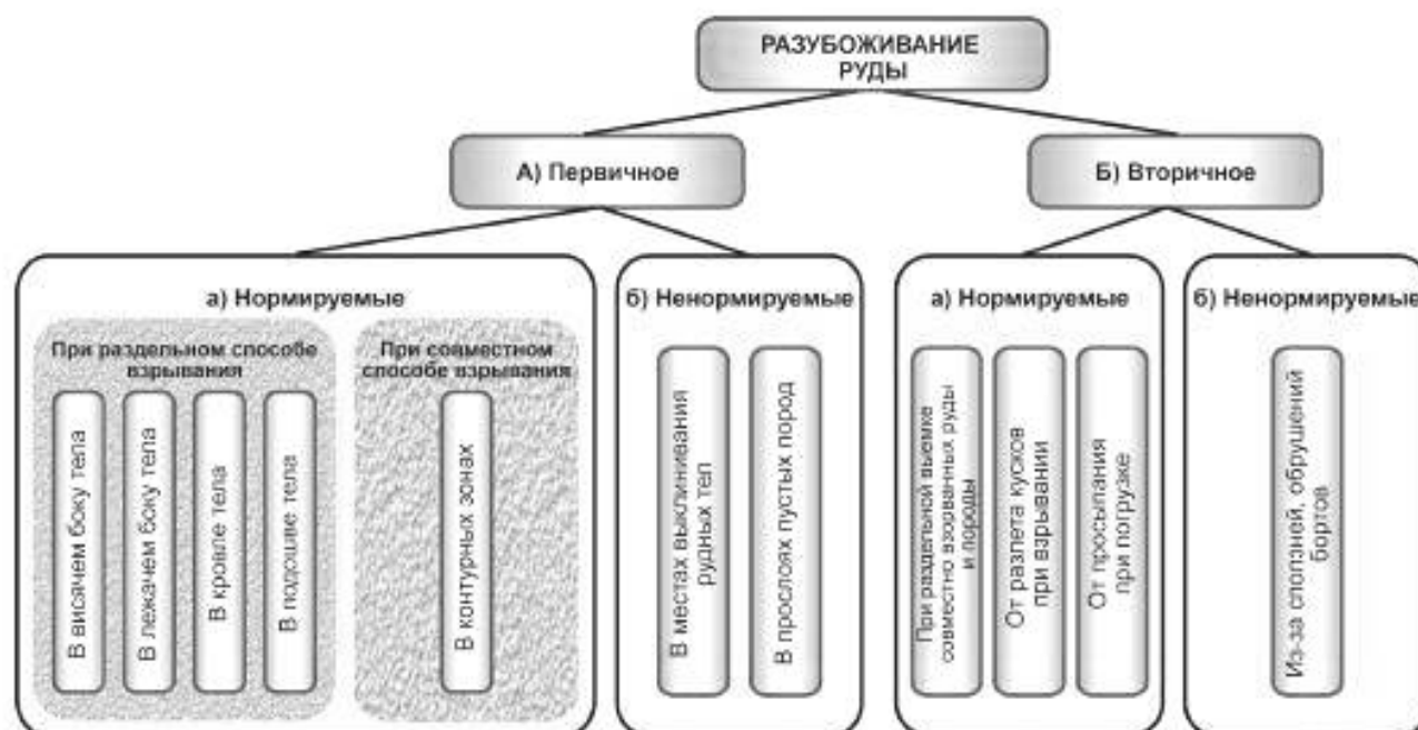
Рисунок 2 — Структура разубоживания алмазосодержащих руд
