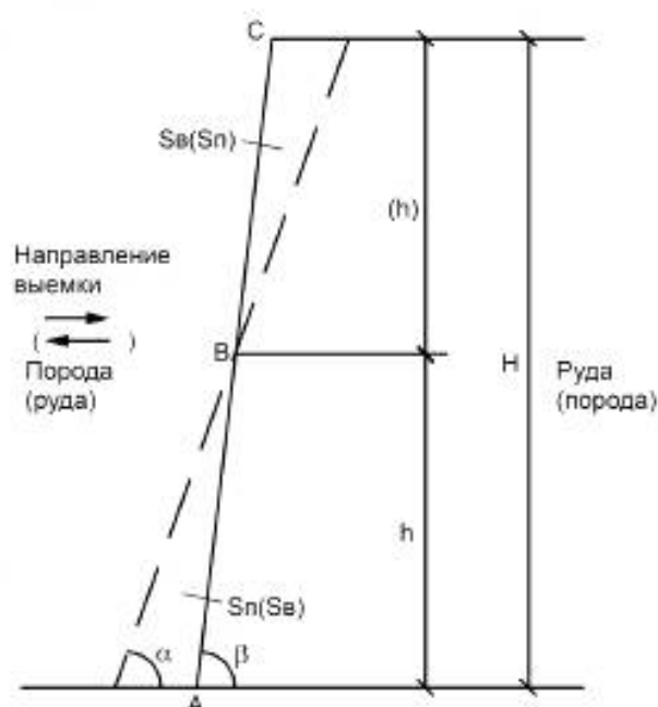
Рисунок 3 — Схема к расчету нормативов потерь и разубоживания руды
