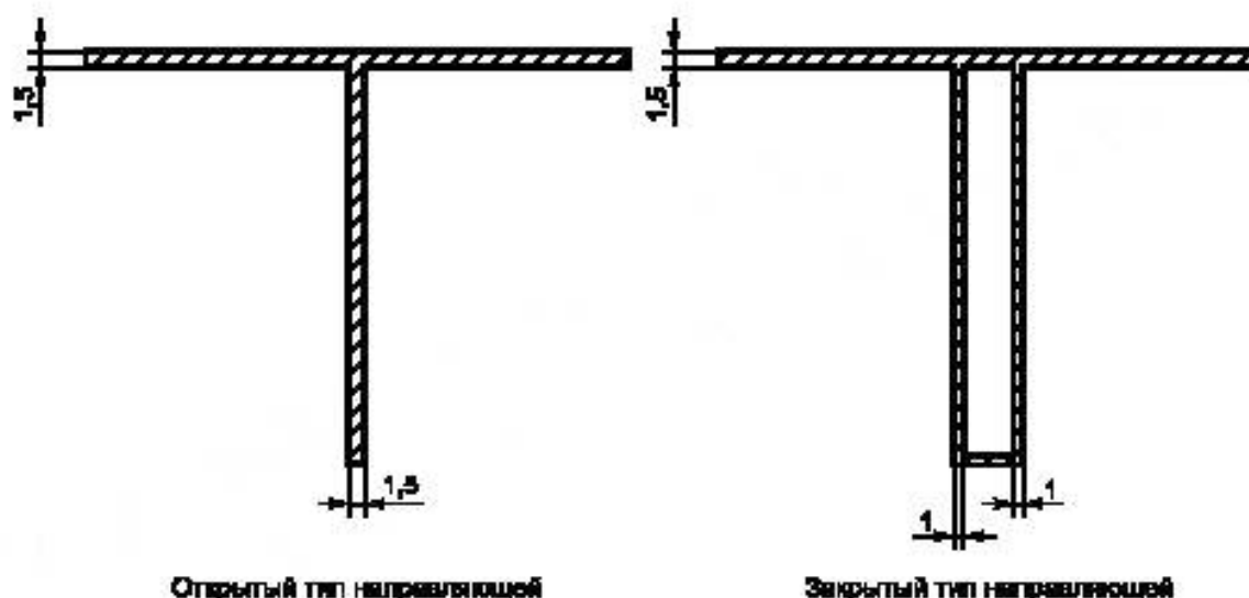
Рисунок 1 — Типы направляющих из алюминиевых сплавов
